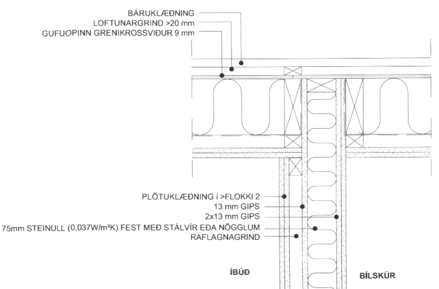
D4 DEILI - EI60 VEGGUR AD ÚTVEGG 1:10
