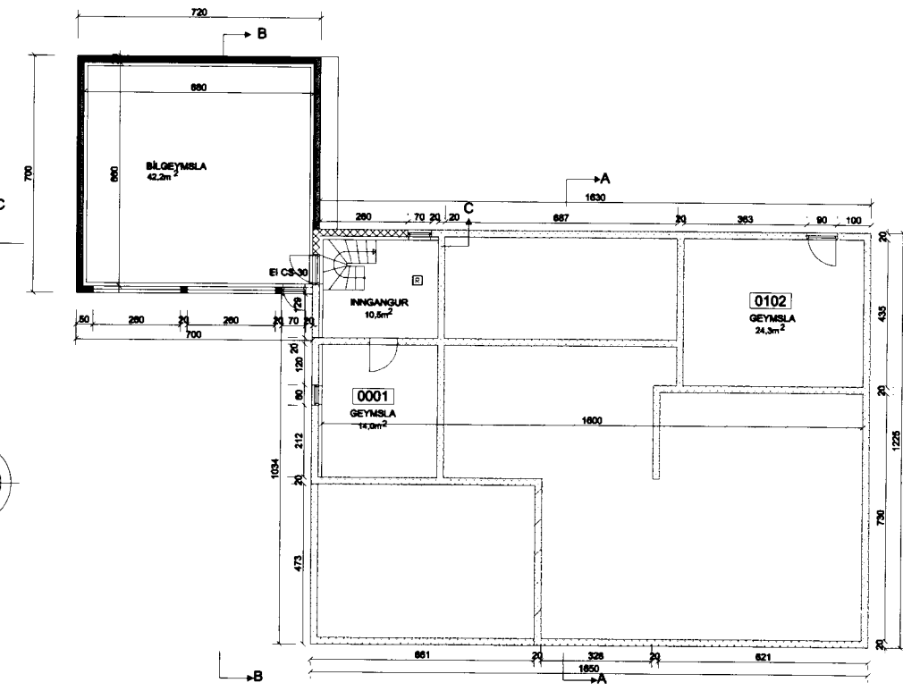
GRUNNMYND KJALLARI
