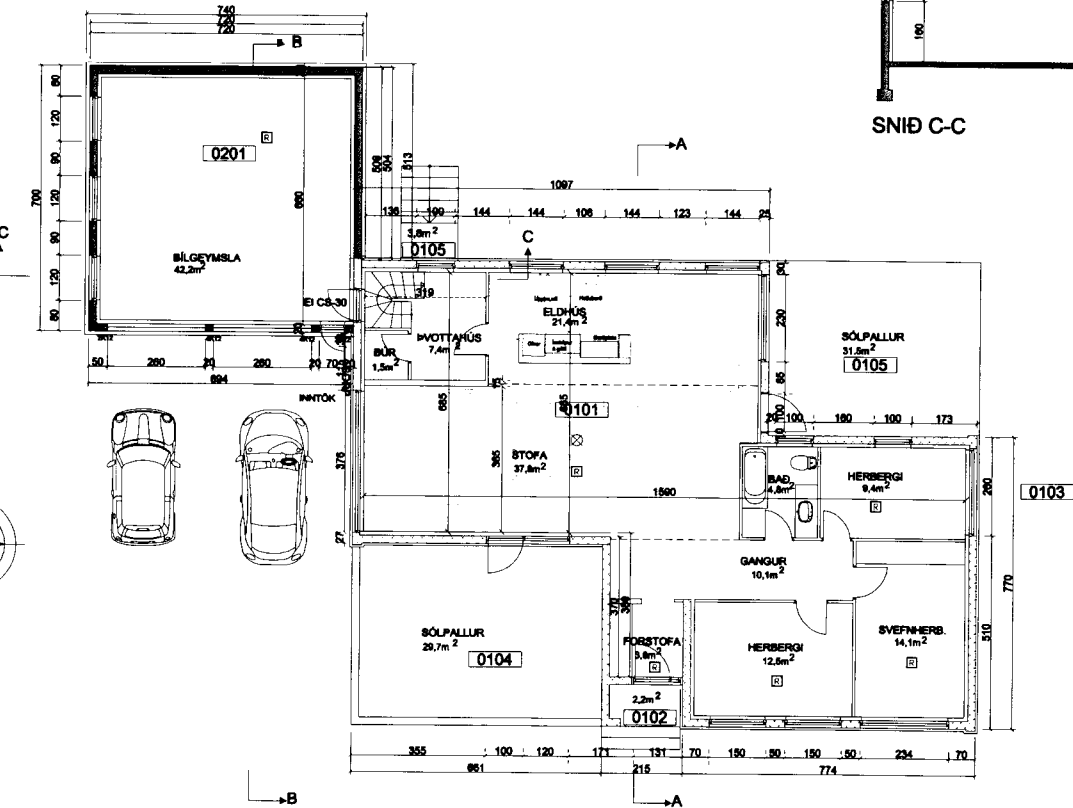
GRUNNMYND 1 HÆÐ
