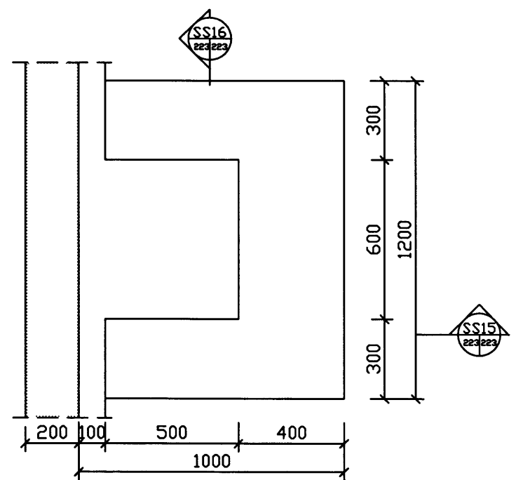
GRUNNMYND VIÐ TENGI BYGGINGU HLÍÐAR
