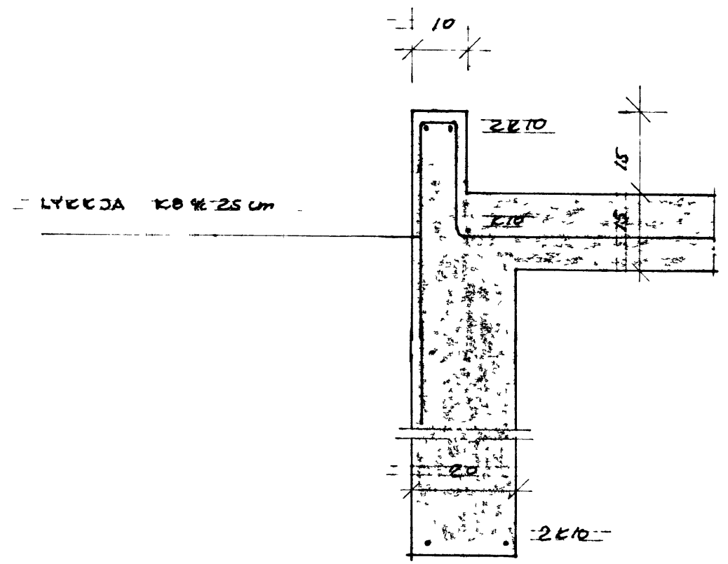
SNID A-A 1/10
