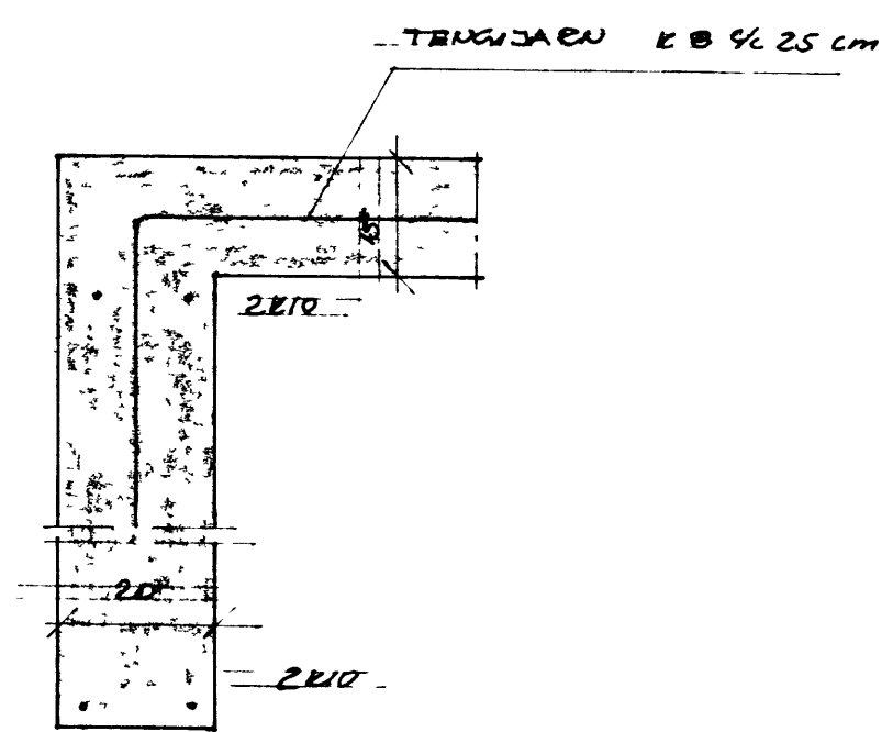
SNID B-B 1/10
