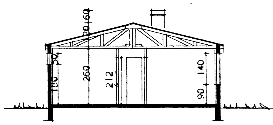
SNEIÐING A--A
