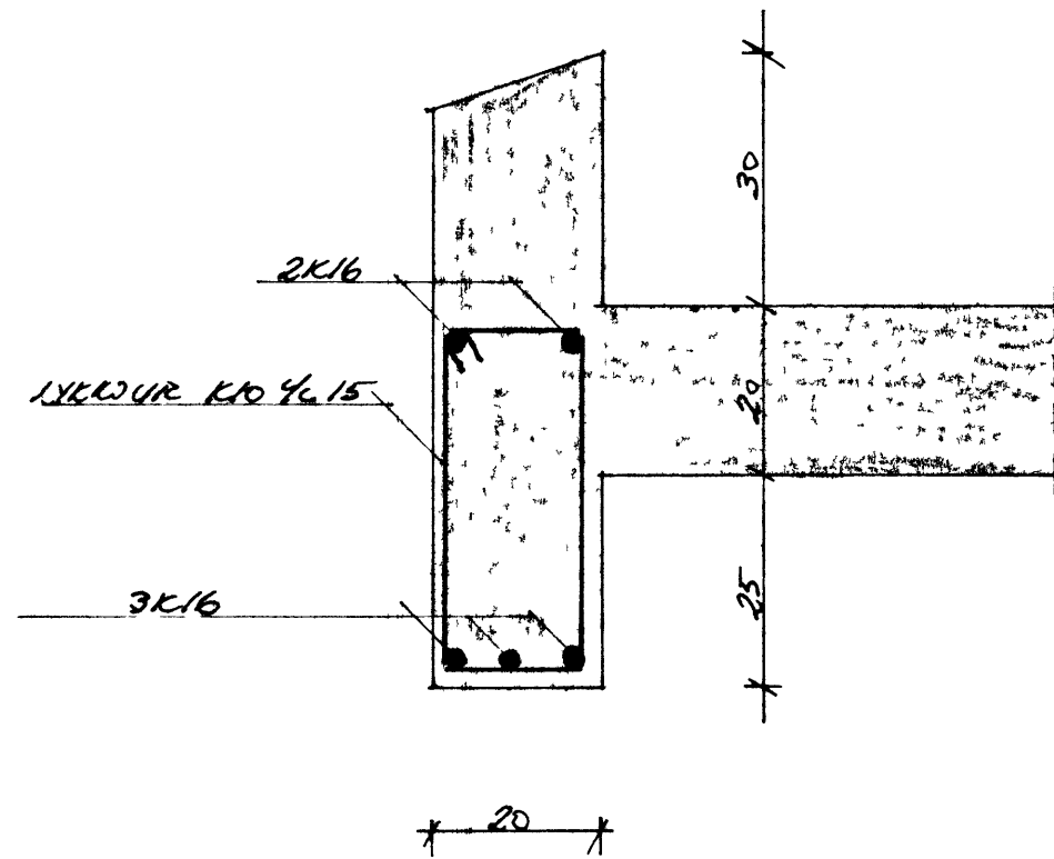
SNID A-A 1:10
