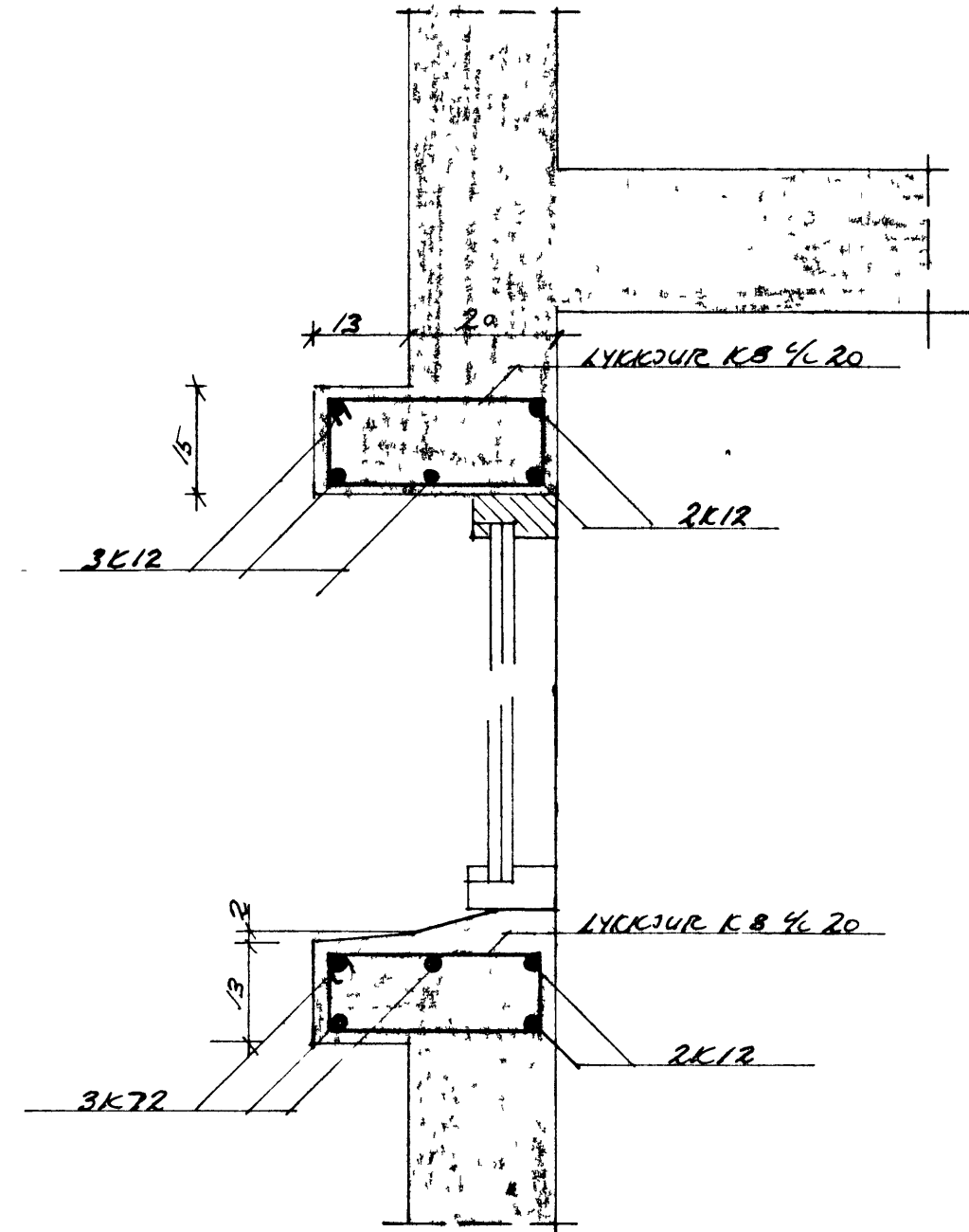
SNID D-D 1:10
