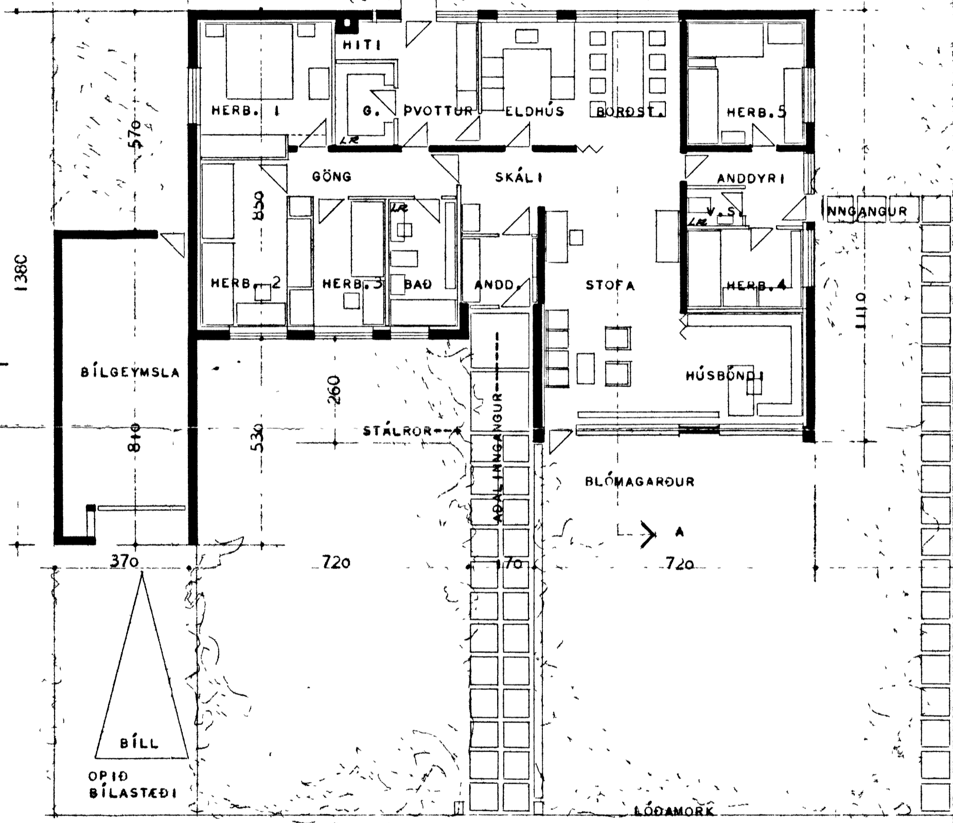
GRUNNMYND
