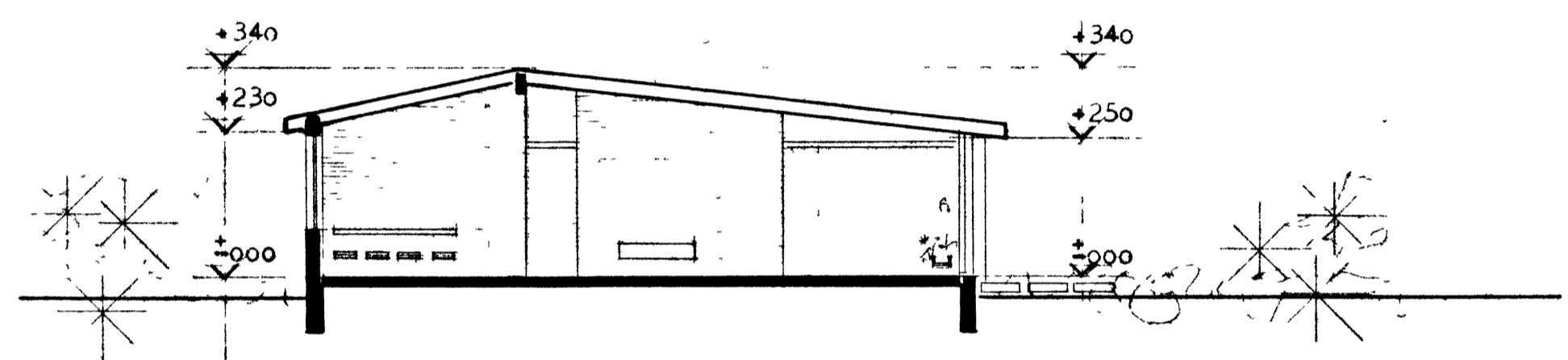
SNEIÐING A-A
