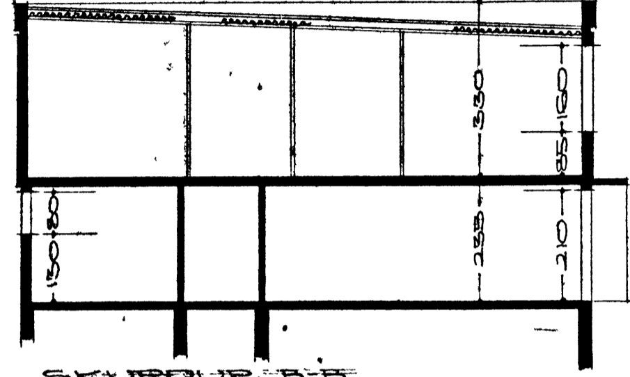
SKURÐUR B-B
