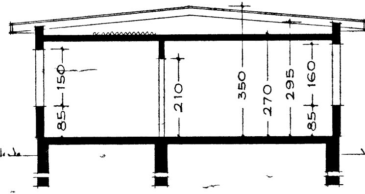
SKURÐUR B-B
