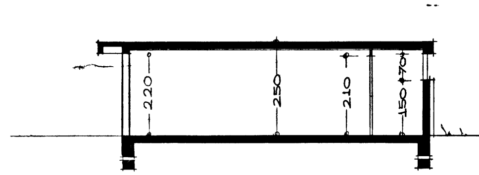
SKURÐUR C-C
