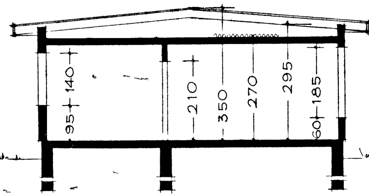
SKURÐUR A-A
