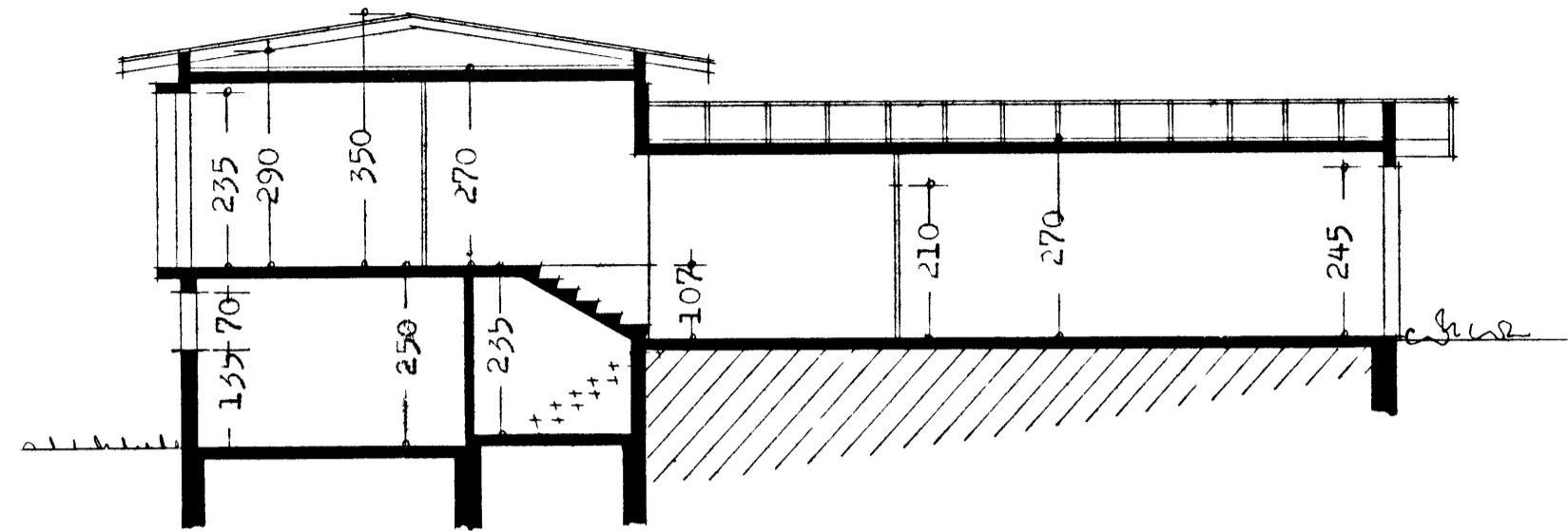
SKURÐUR A-A
