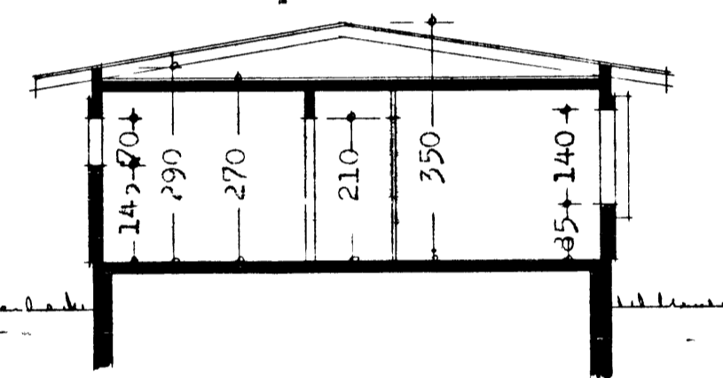
SKURÐUR B-B
