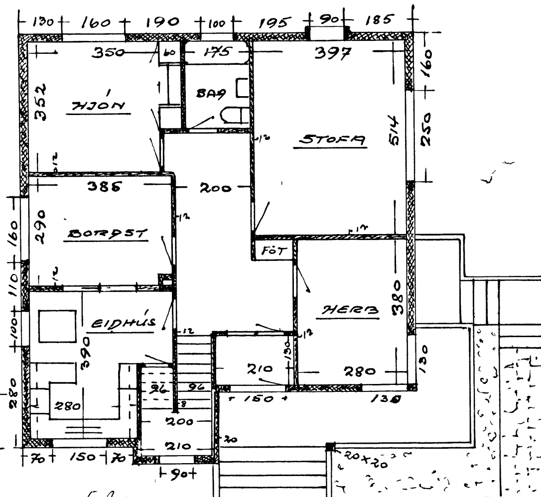
1 HÍÐ
