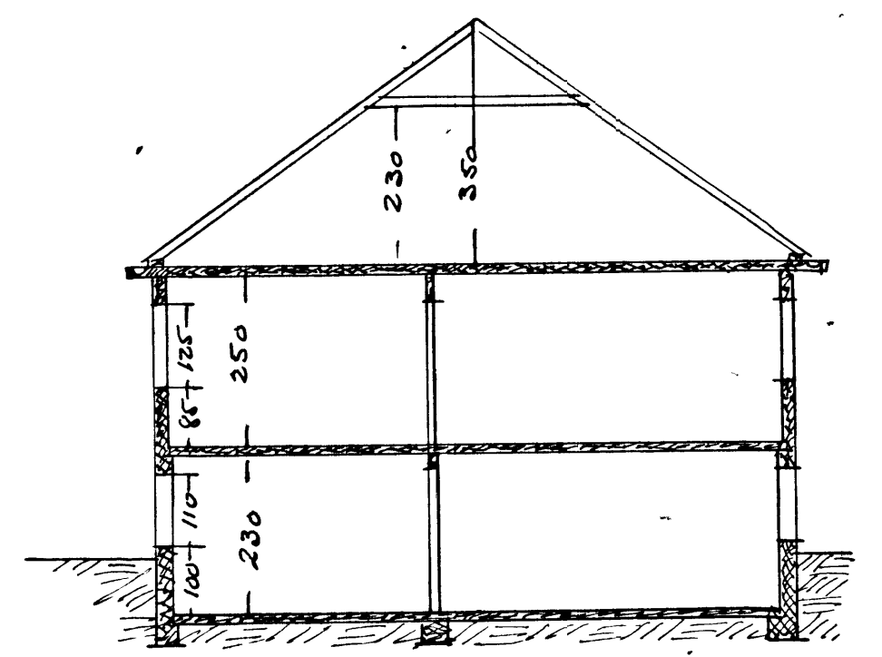
SKURÐUR
