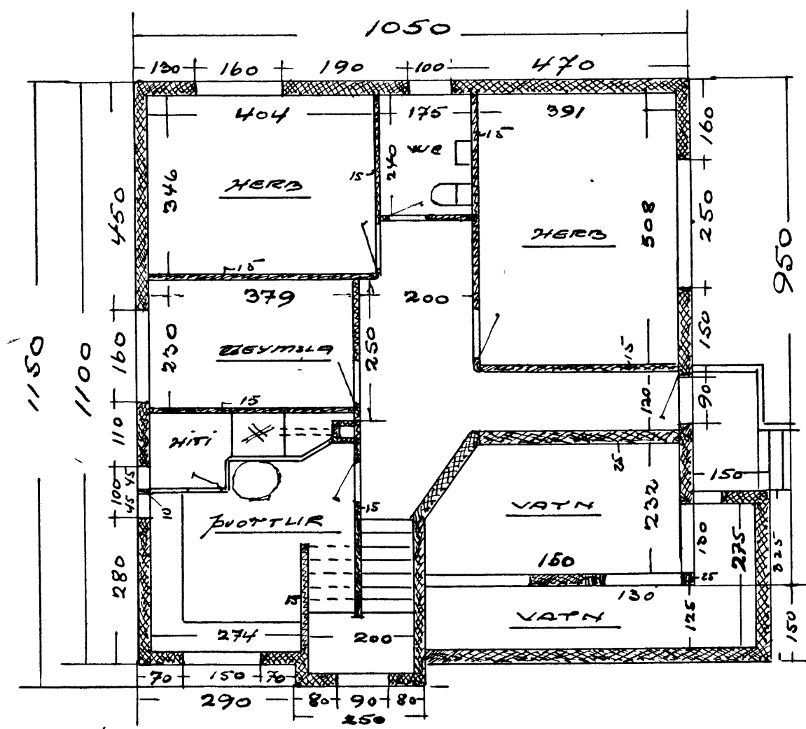
KJALLARI
