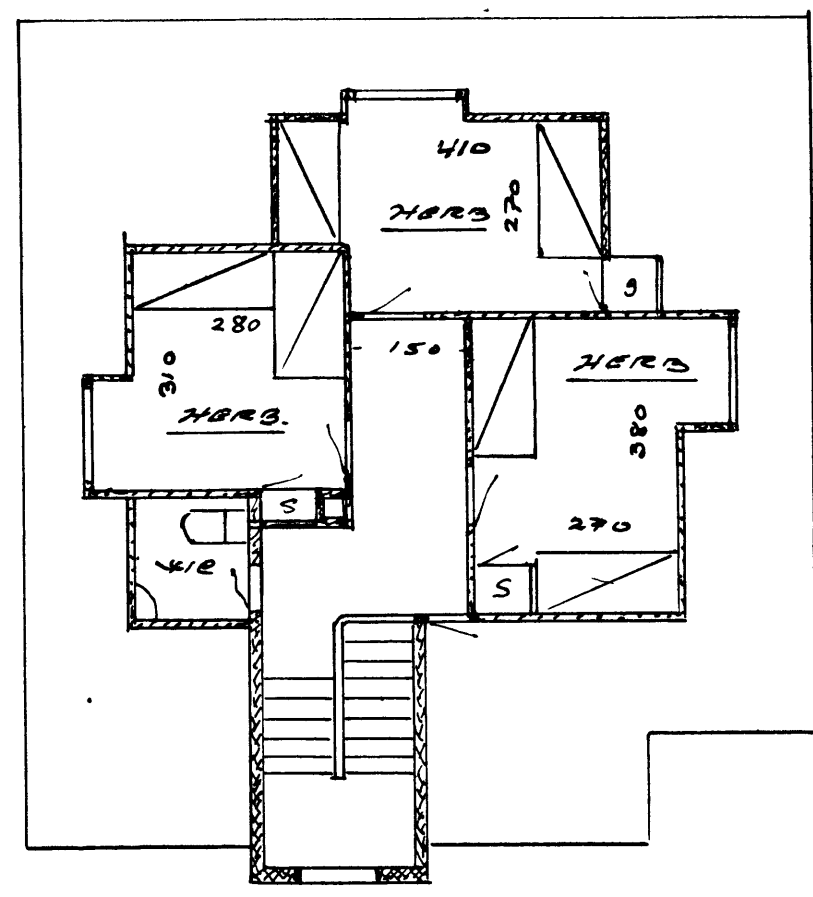
ÞAKHÍÐ
