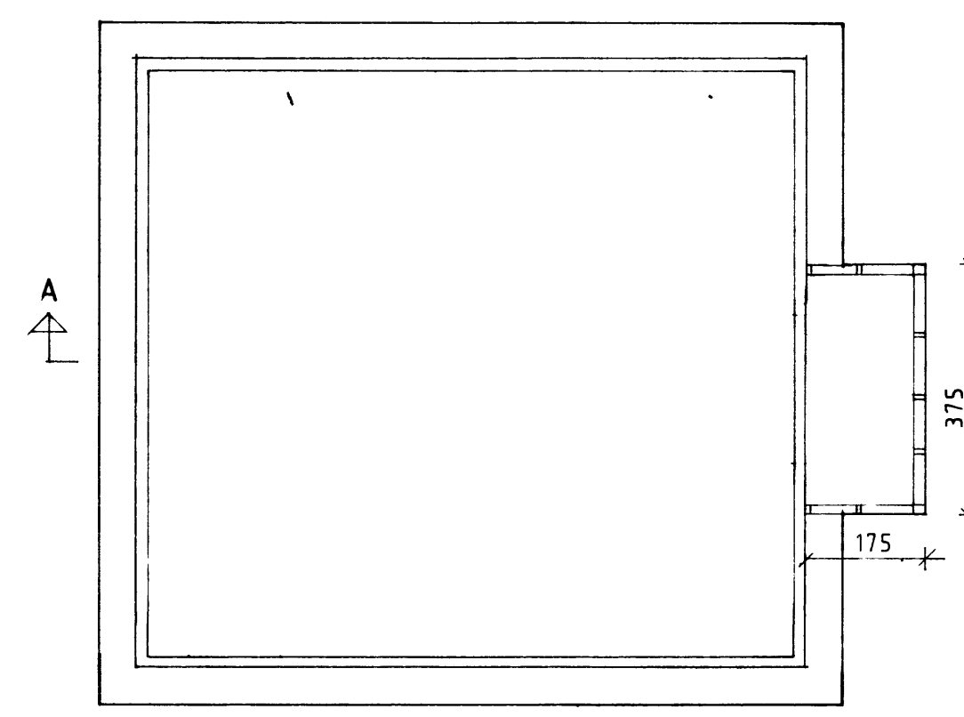
GRUNNMYND ÞAK
