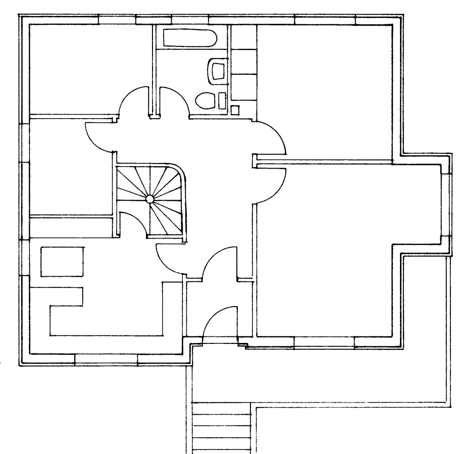
GRUNNMYND 1 HÆÐ
