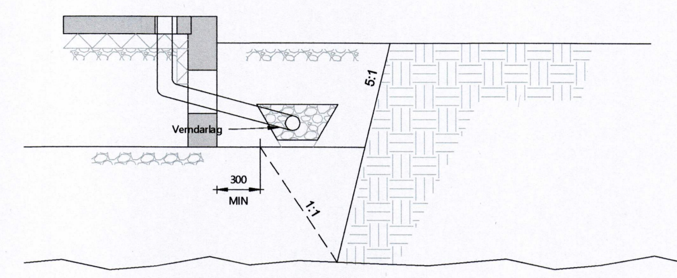
Snið í sökkli 1:25
