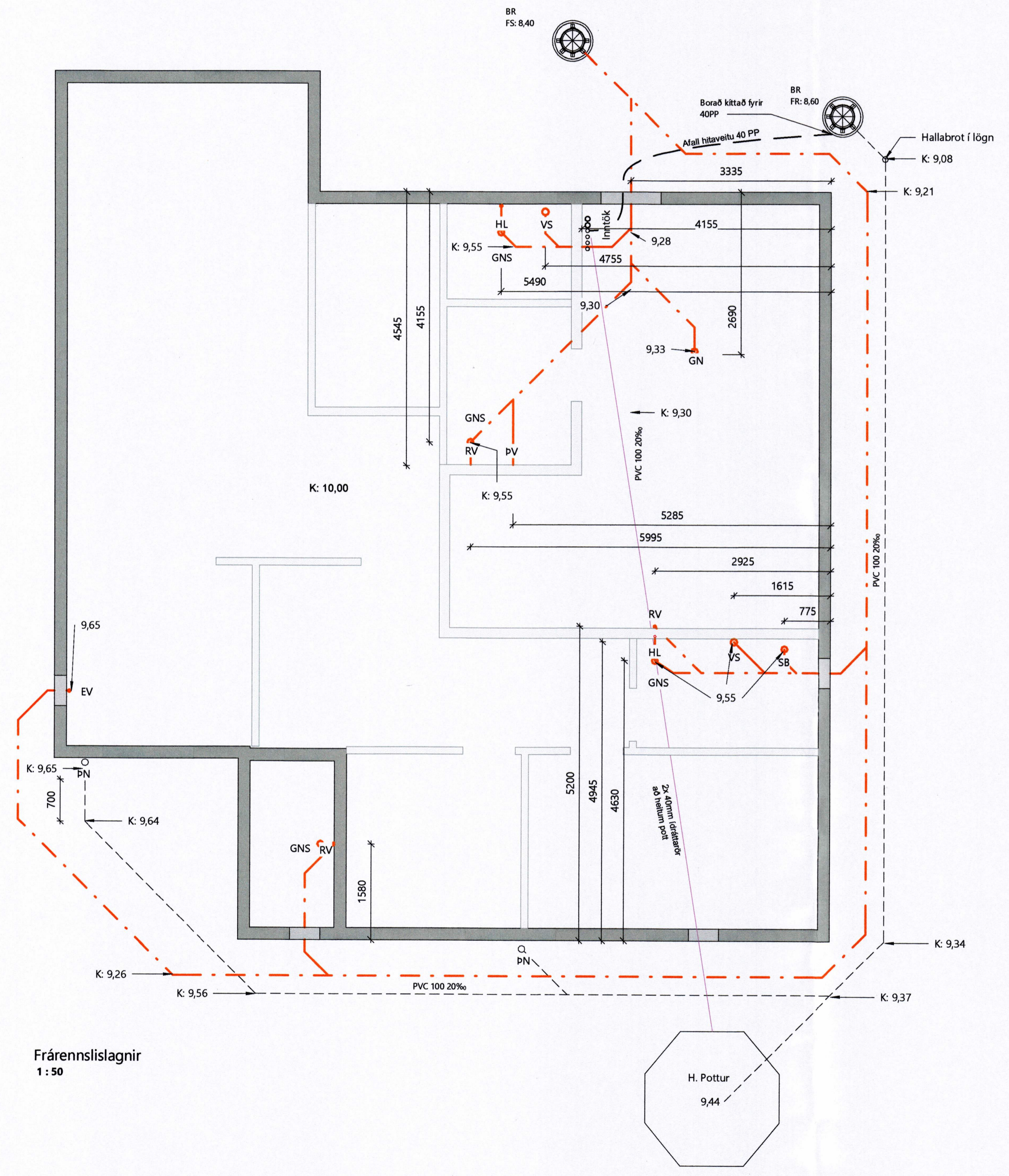
Skýringar Kótar 1:10
