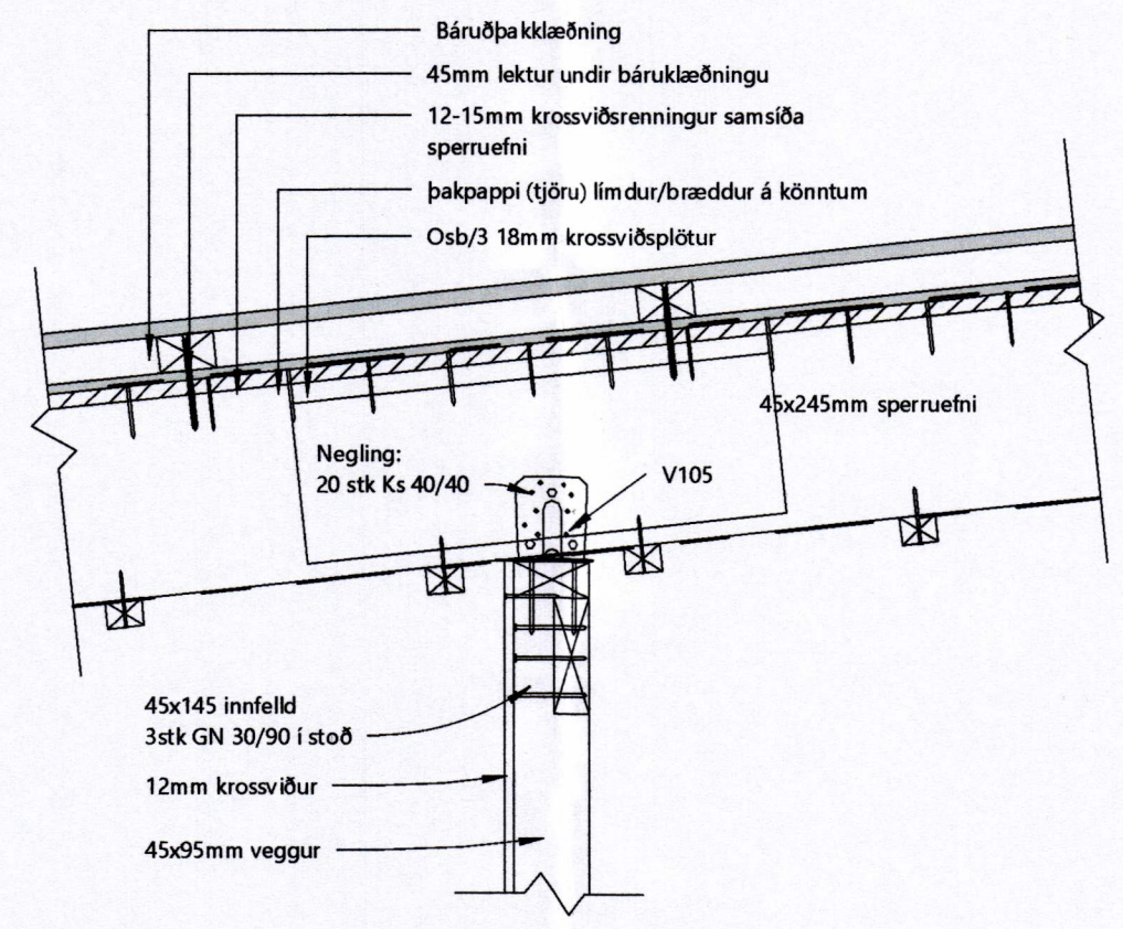
D20 Veggur Pak Frágangur 1:10
