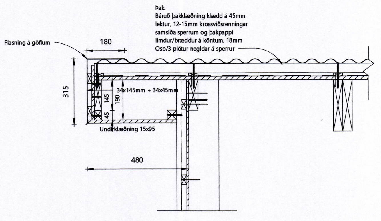
D10 Pakkantur stafnar 1:10
