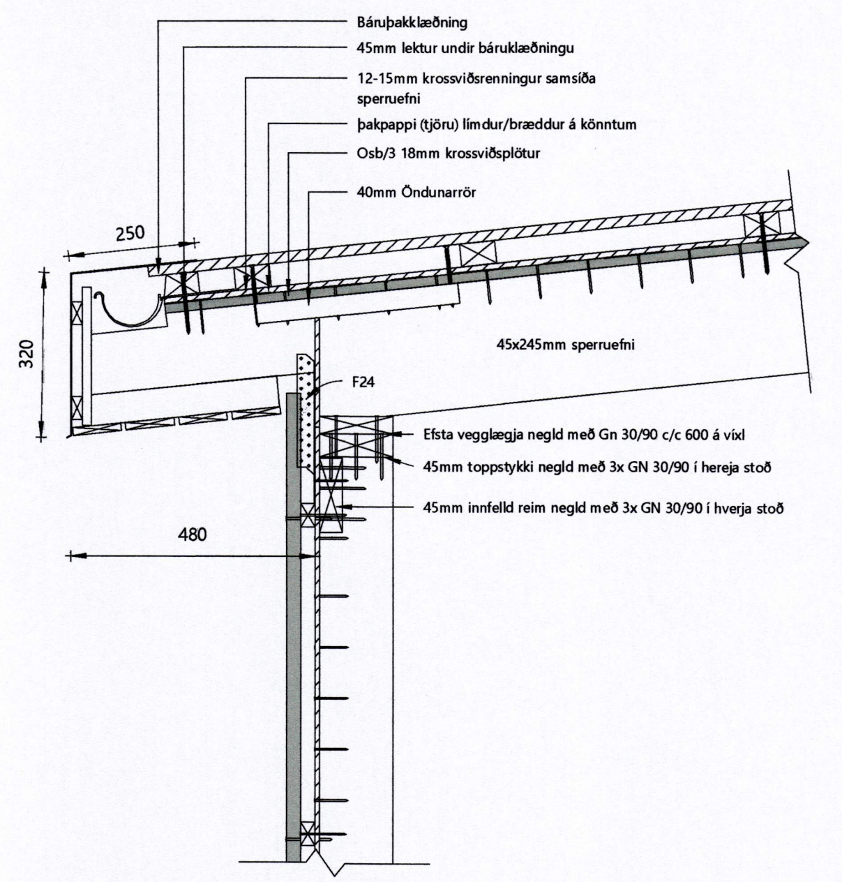
D7 Pakkantur frágangur Renna inn í kannti 1:10
