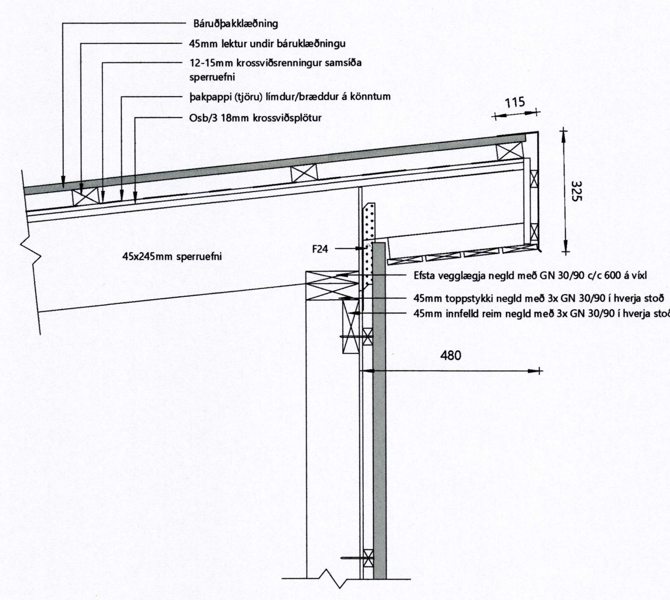
D24 Pakkantur útveggur 1:10
