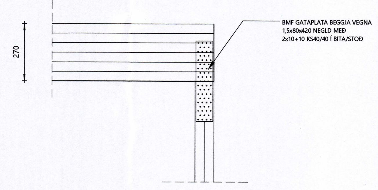
B-FRÁGANGUR BITA VIÐ SÚLUR 1:10
