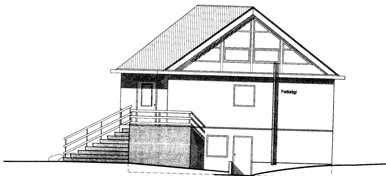
ÚTLIT NORÐUR -eftir breytingu
