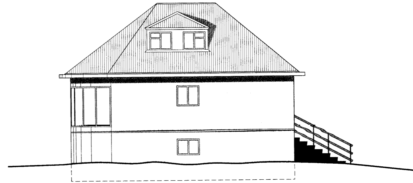
ÚTLIT SUÐUR -fyrir breytingu
