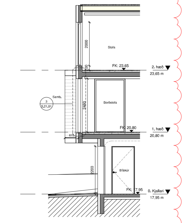
5 Hlutasnið 1 : 50
