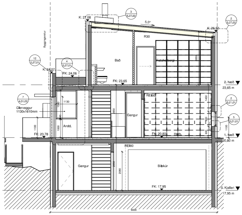
2 Þversnið. 1 : 50
