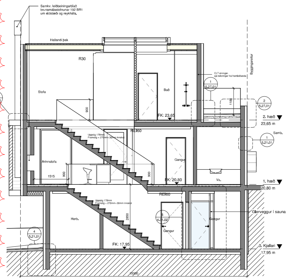
1 Langsnið. 1 : 50
