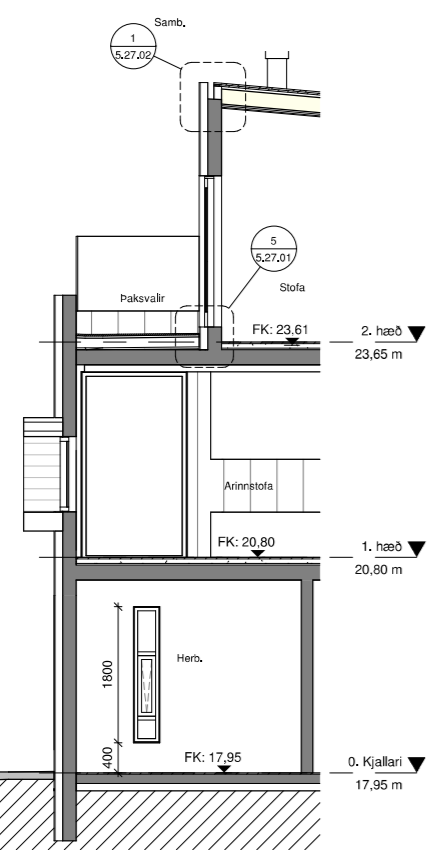
3 Hlutasnið 2 1 : 50
