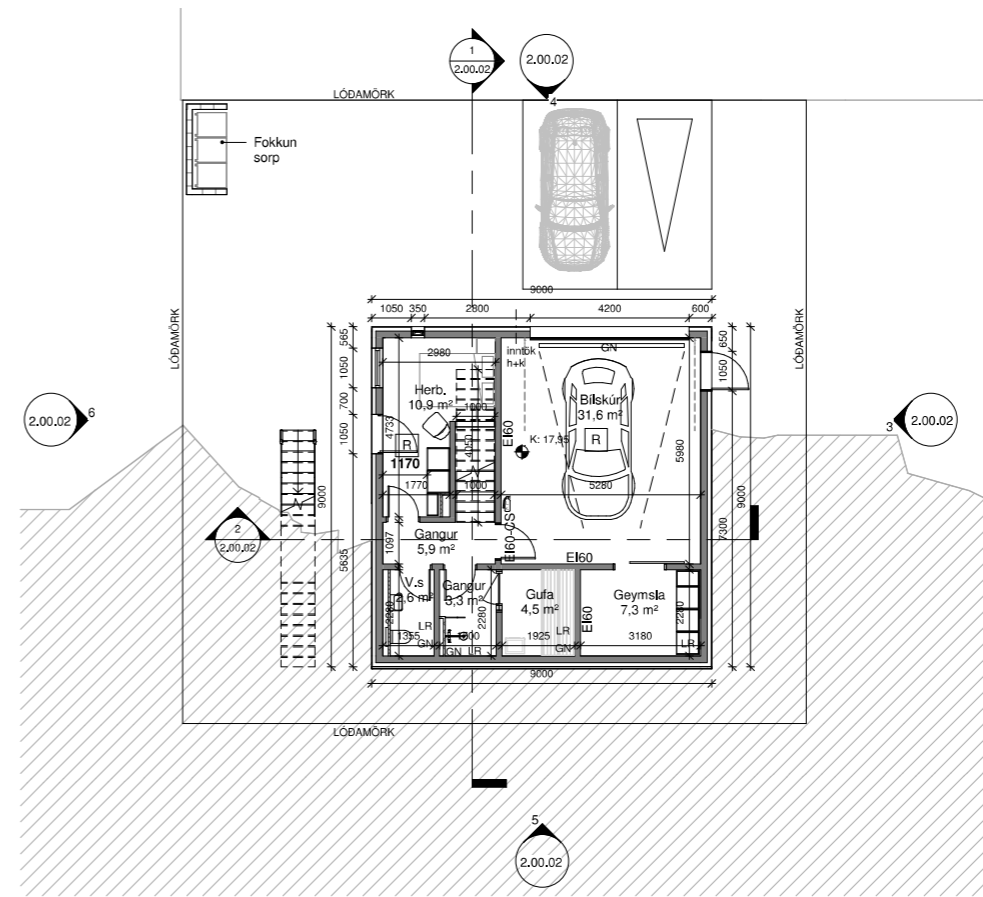
1 0. Kjallari 1 : 100
