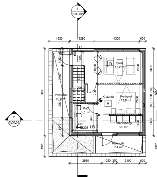
3 2. hæð 1 : 100
