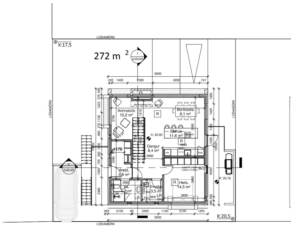
2 1. hæð 1 : 100
