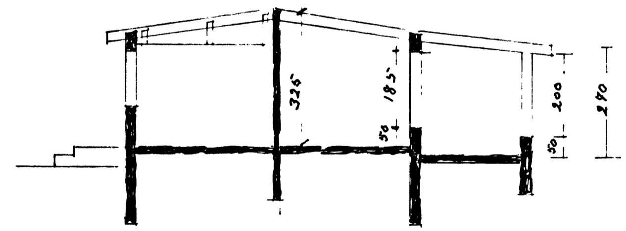
Sneidning
