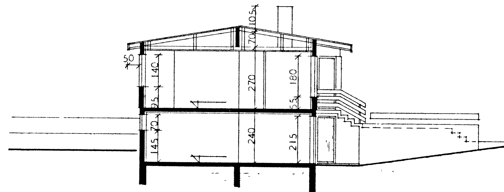
SNEIÐING A-A
