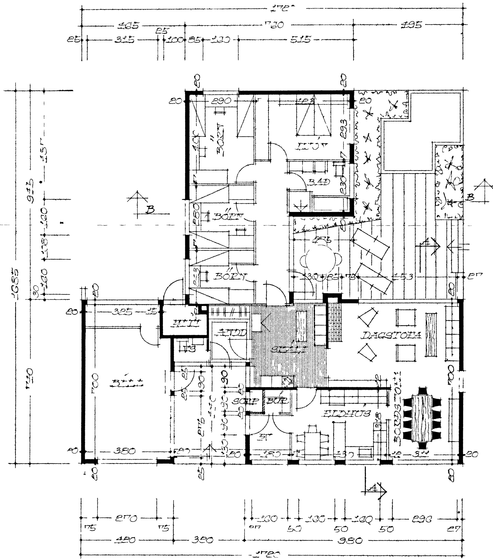
GRUNNMYND
