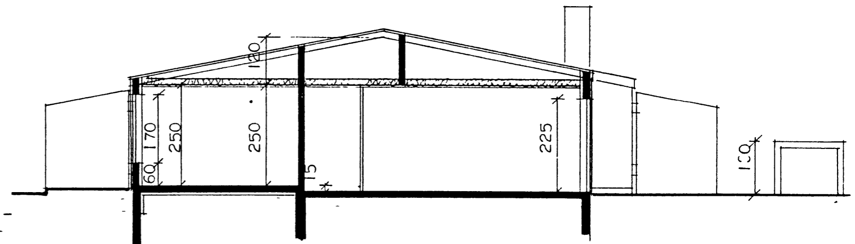
SNEIÐING A-A 1:100
