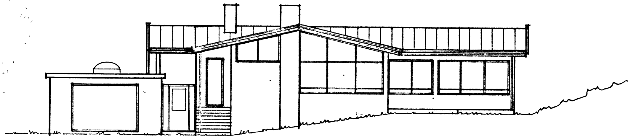
SUÐURHLID 1:100
