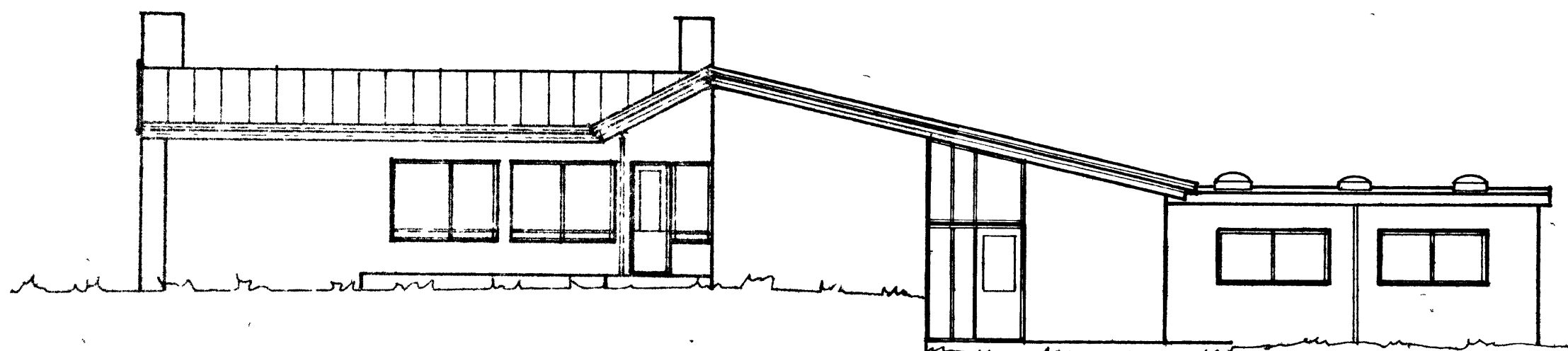
AUSTURHLID 1:100
