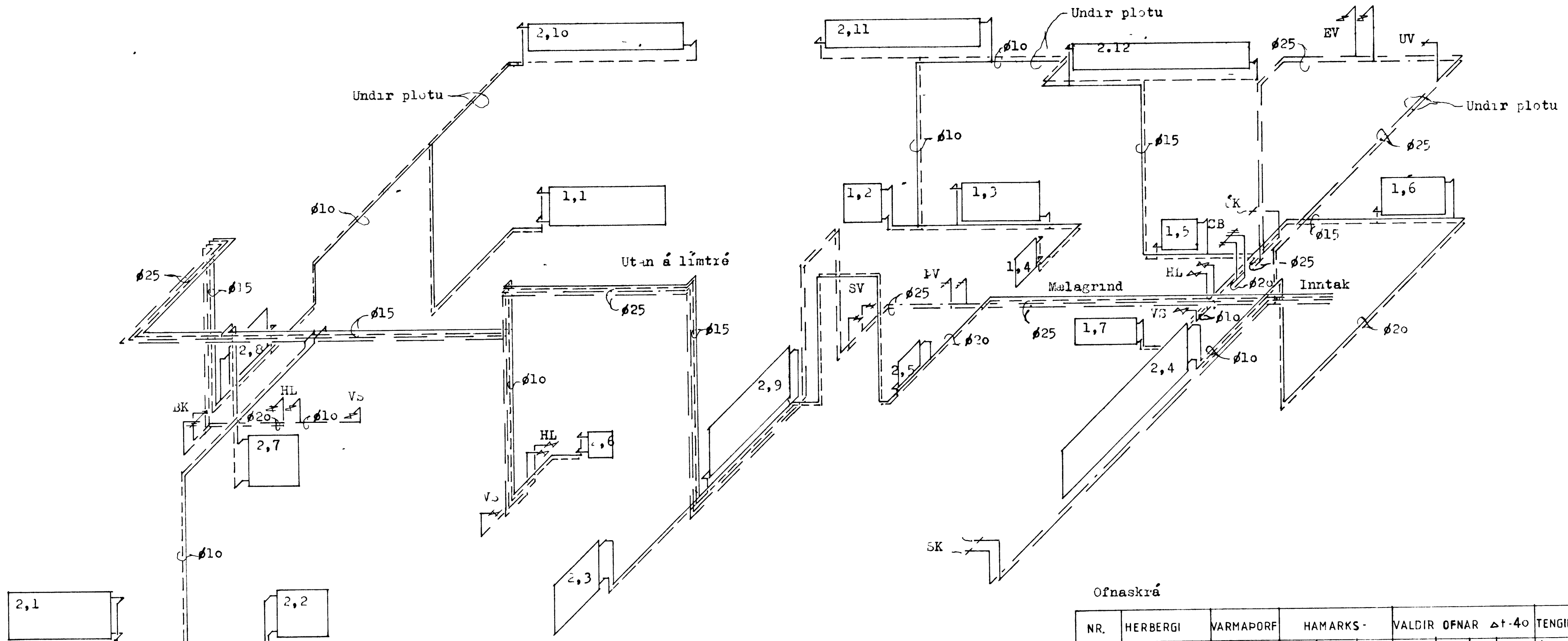
Rúmmynd 1:50
