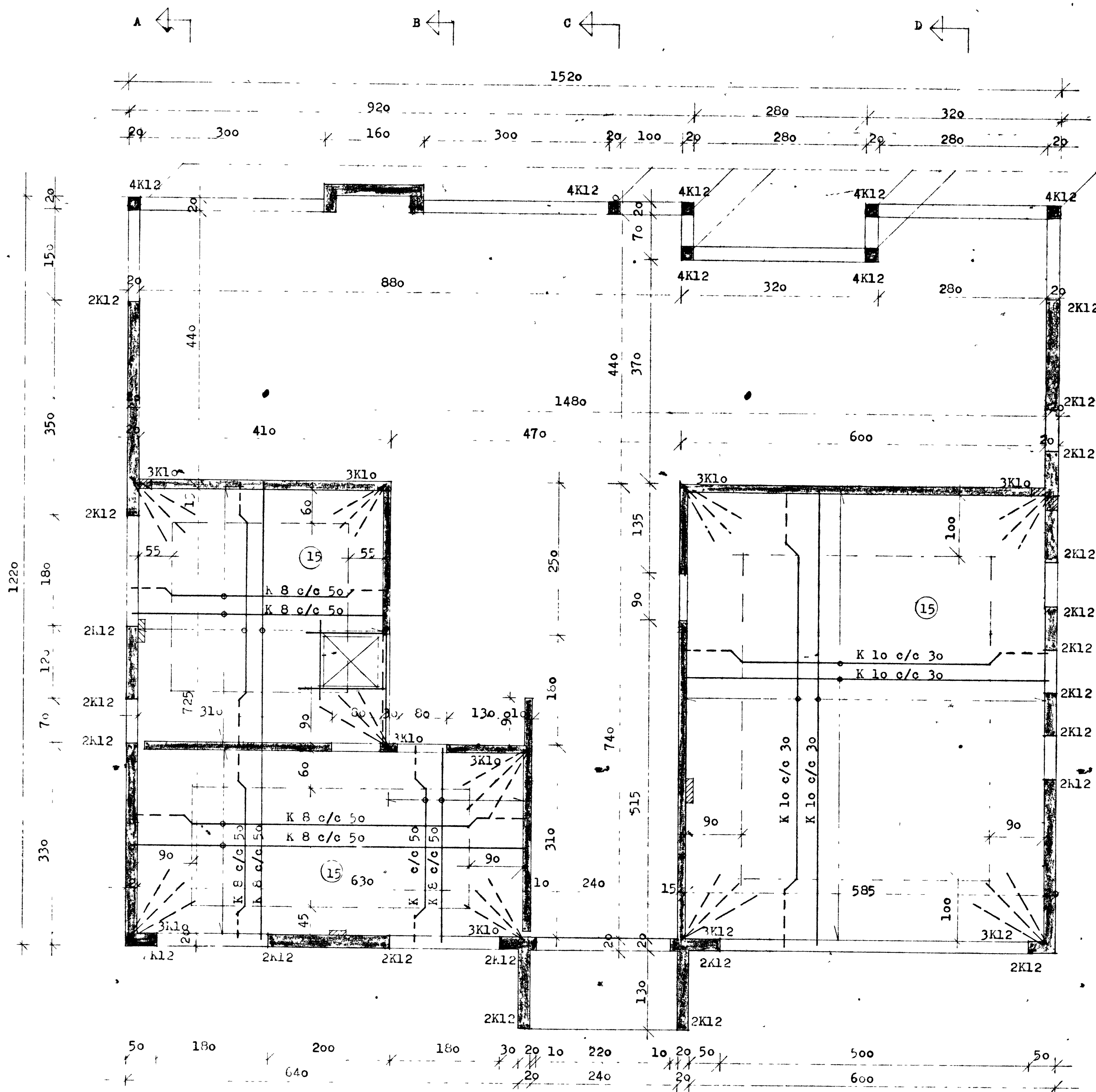
Grunnmynd 1 hæð 1:50
