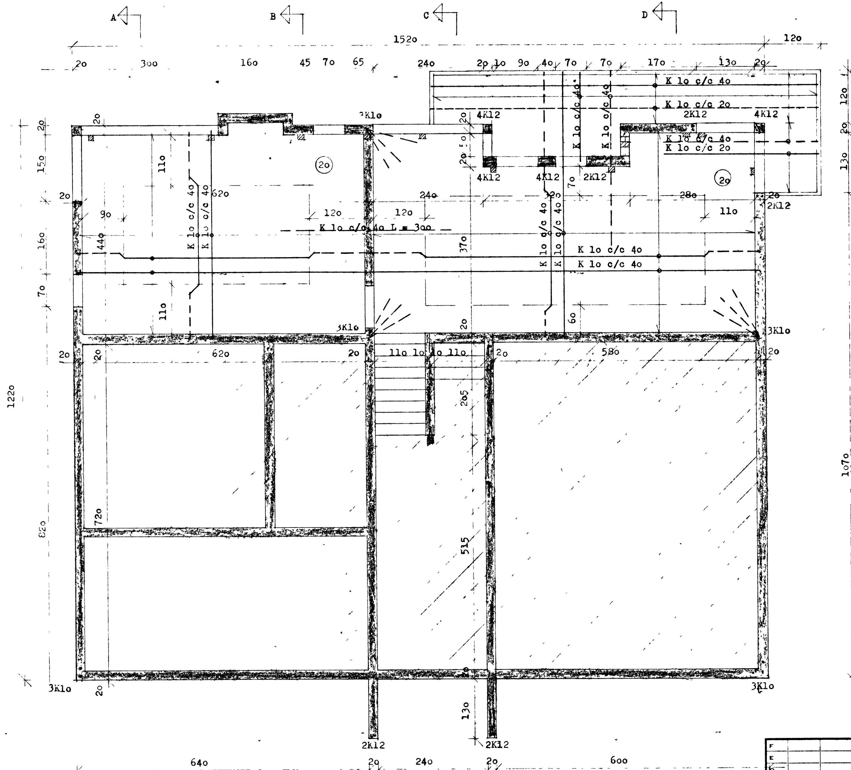
Grunnmynd kjallari 1:50
