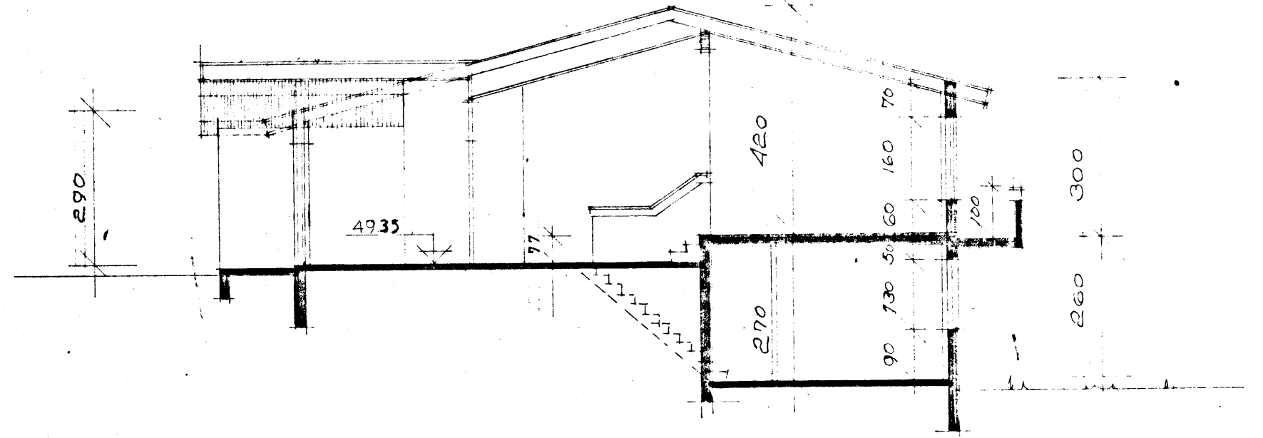
ÞVEÐSNID 1:100
