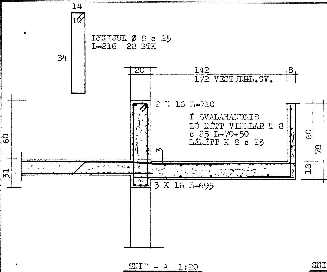
SNIE - A 1:20
