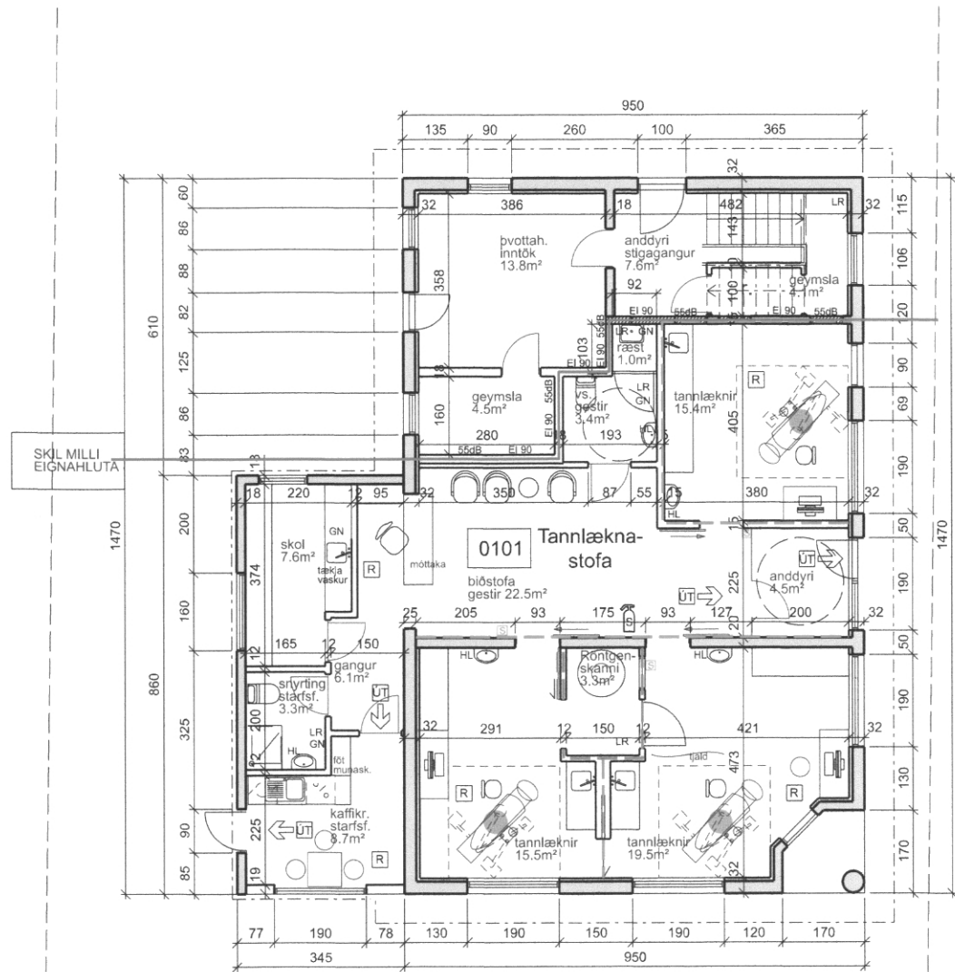
1 GRUNNMYND 1:100 10-02 GRUNNMYND 1 HÆÐAR / breyting
