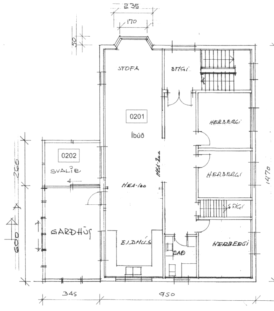
2 GRUNNMYND 1:100 10-02 GRUNNMYND 2 HÆÐAR / teikn. Páll Z.
