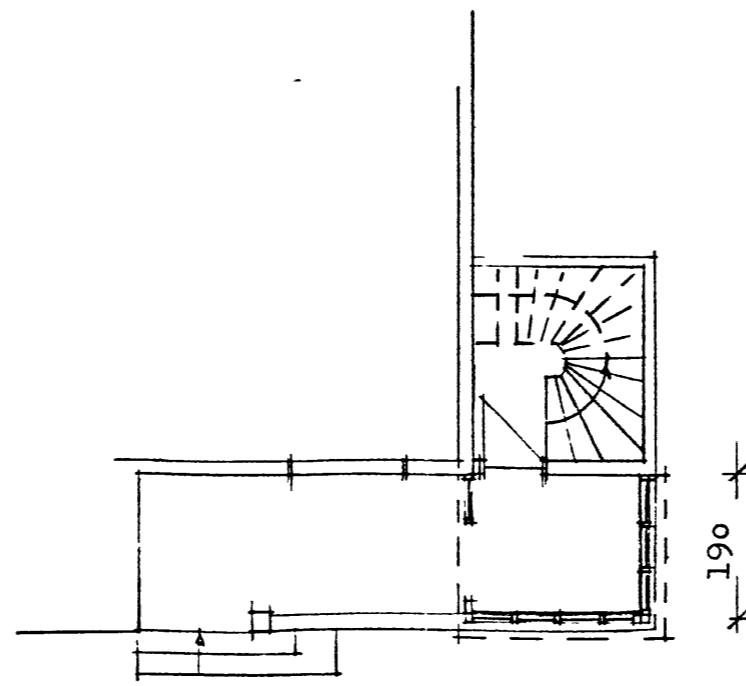
GRUNNMYND
