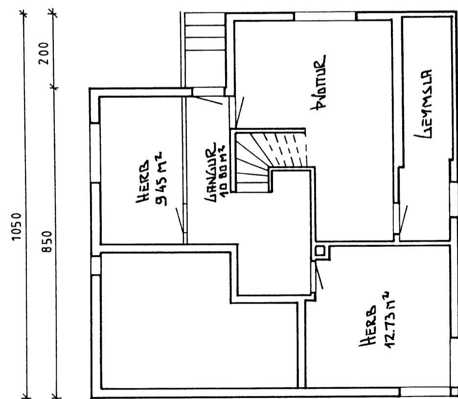
KJALLARI
