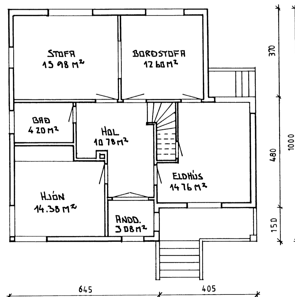
1 HÆÐ
