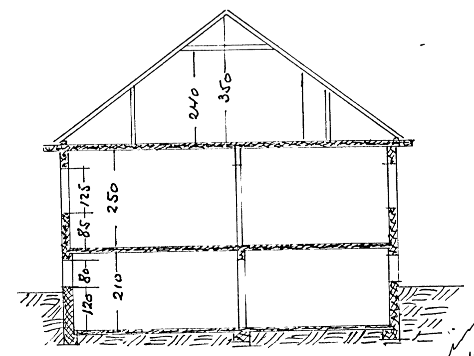
SKURÐUR
