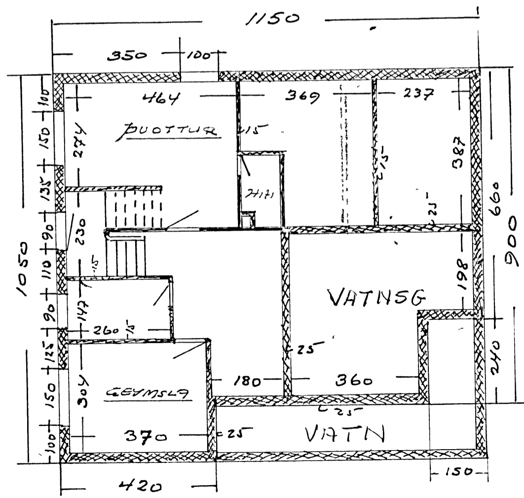
KVALLARI
