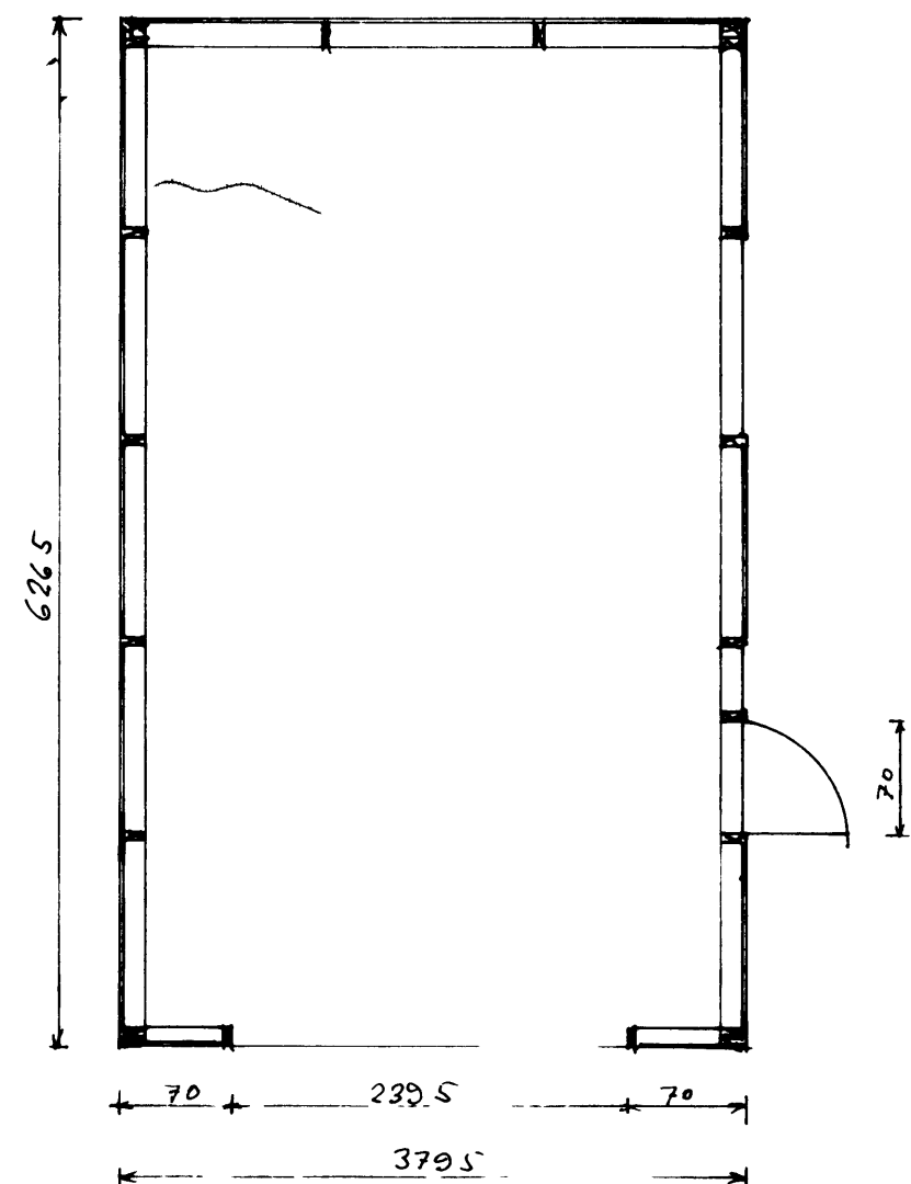
Grunnmynd 1:50
