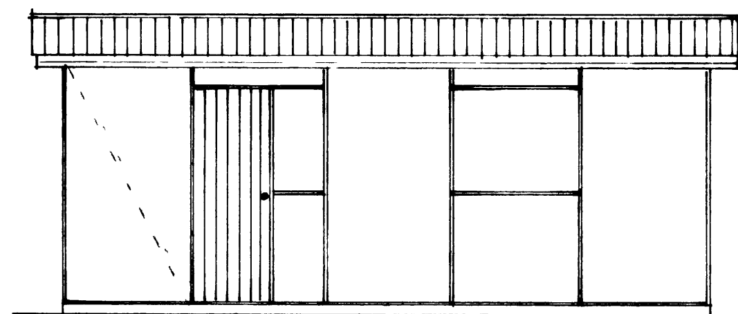
Norður 1:50
