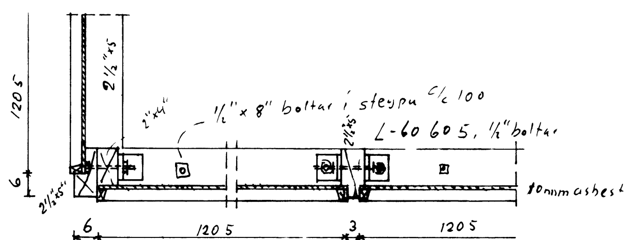
Lárrétt sniðing 1:10
