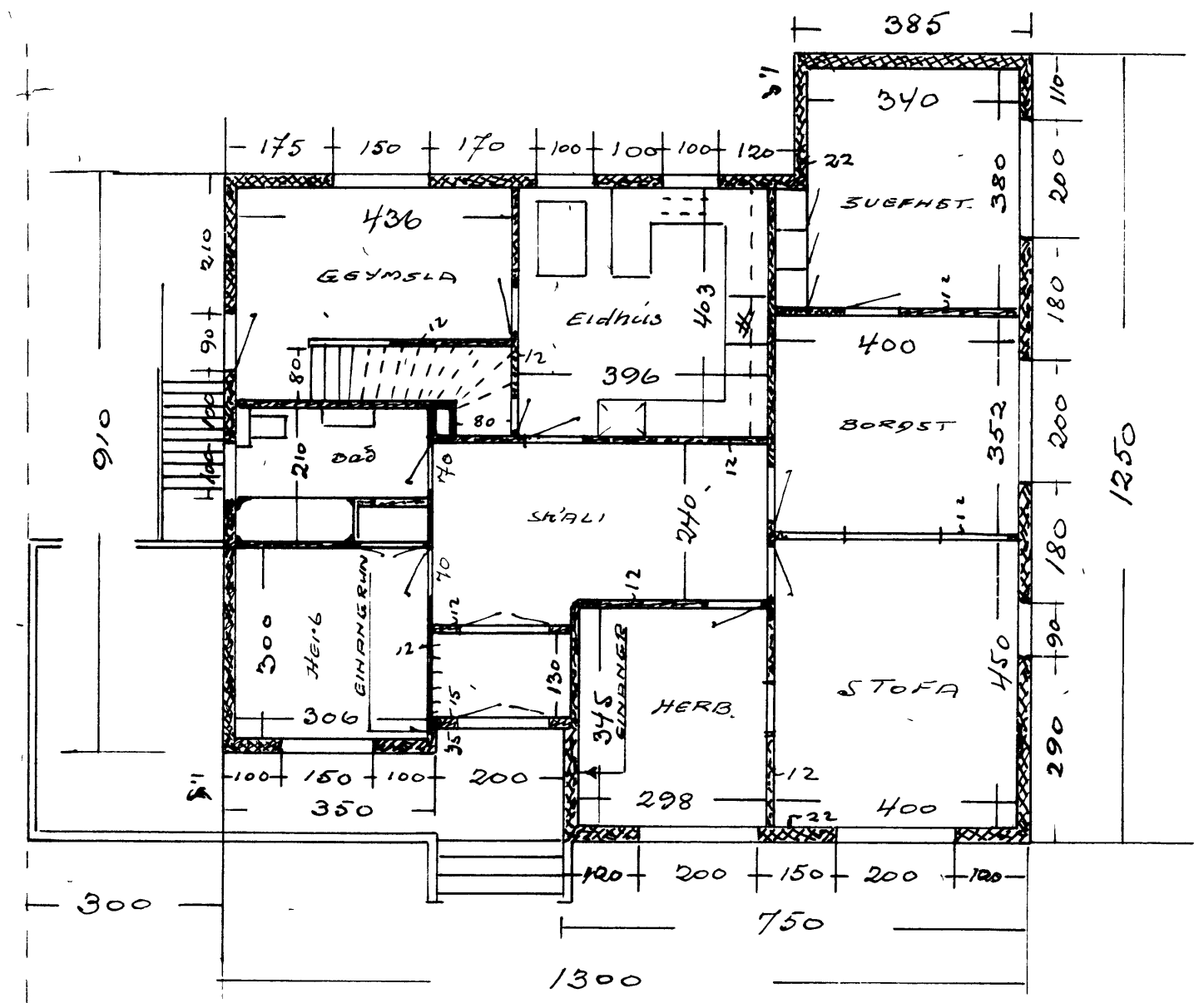
1 HÆÐ
