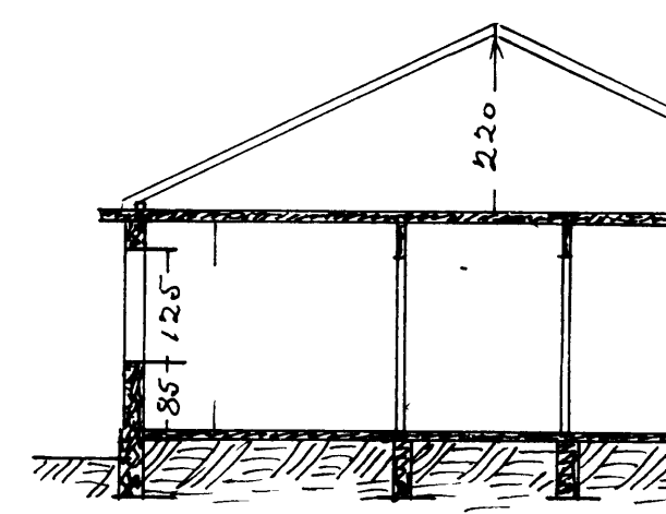
SKURÐUR
