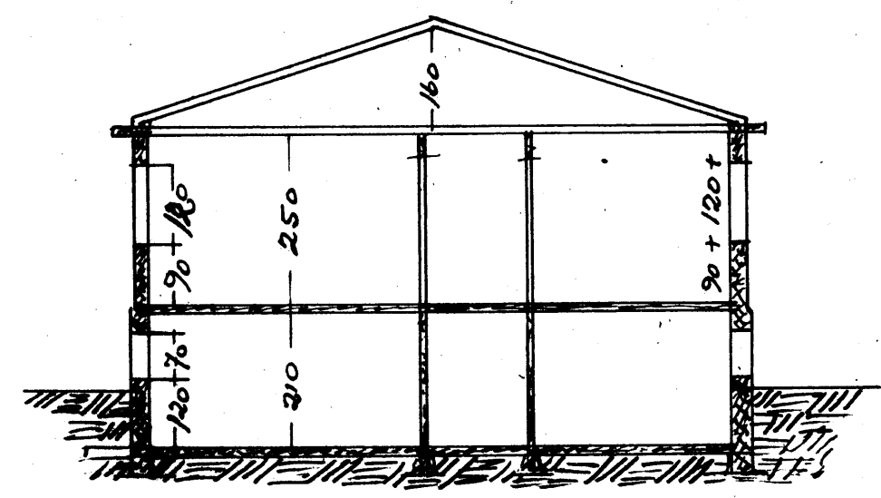
SKURÐUR
