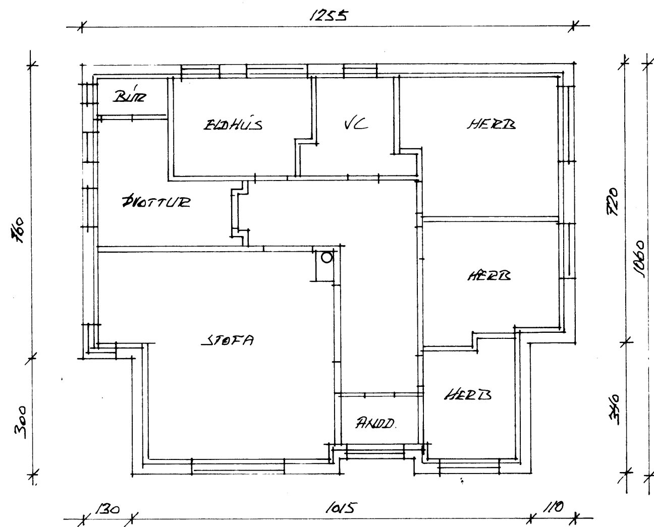
GRUNNMYND
