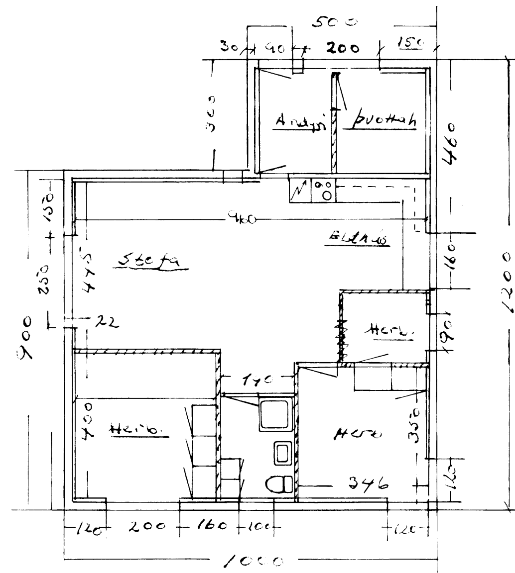
GRUNNFLOTTUR
