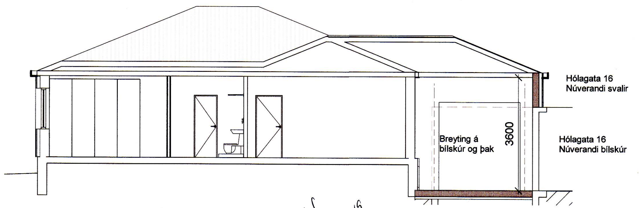
Langsnið A 1 : 100
