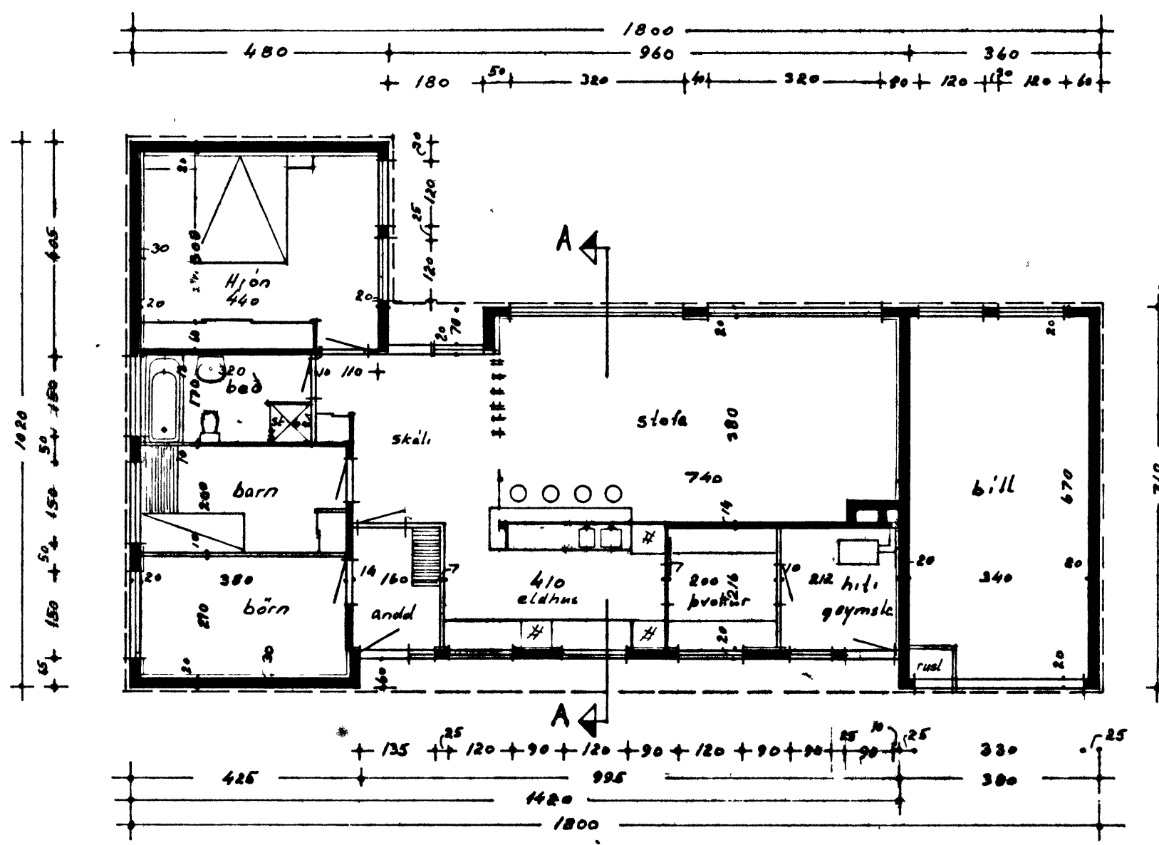
Grundmynd M1:100
