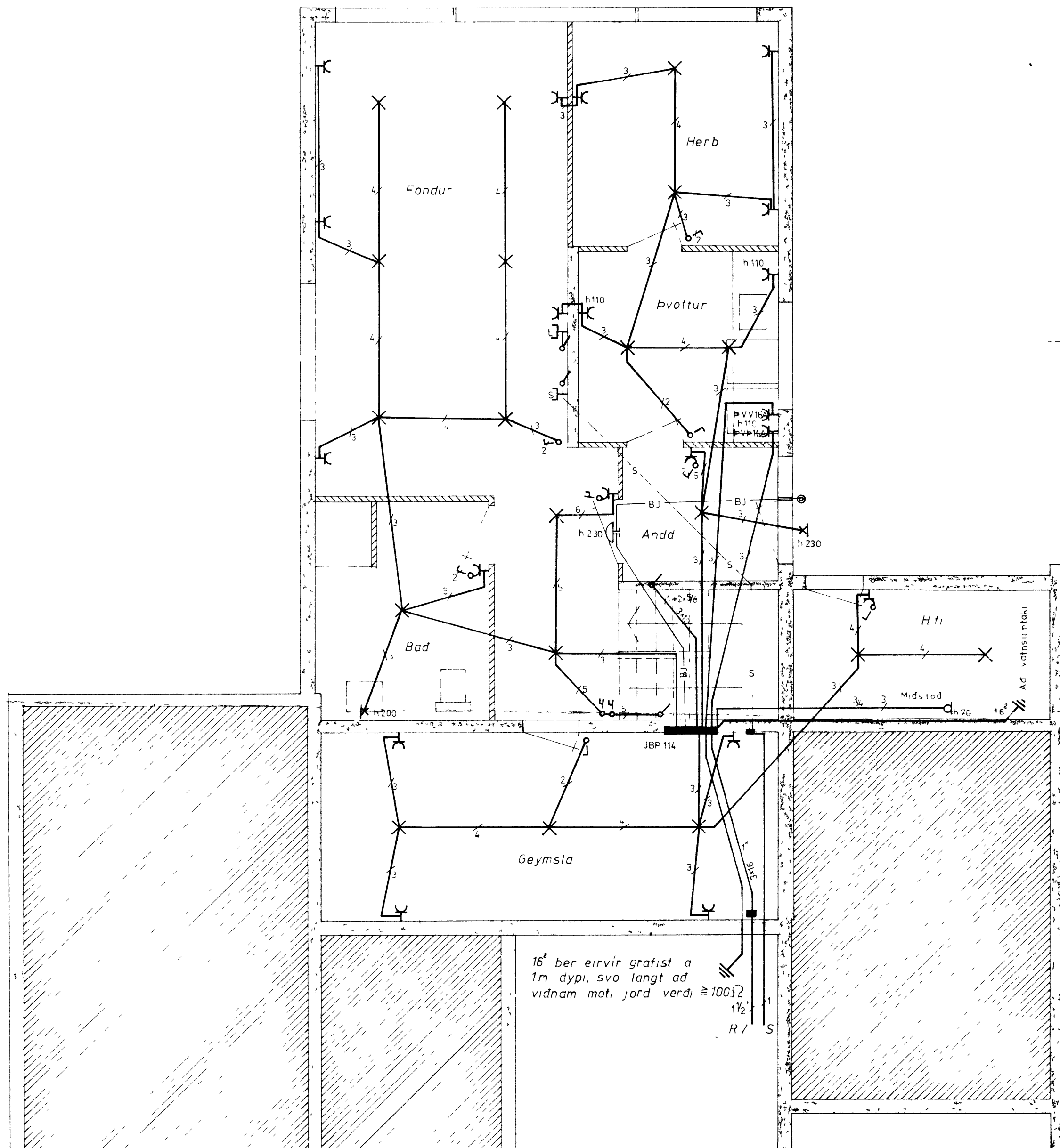
KJALLARI, M=1 50
