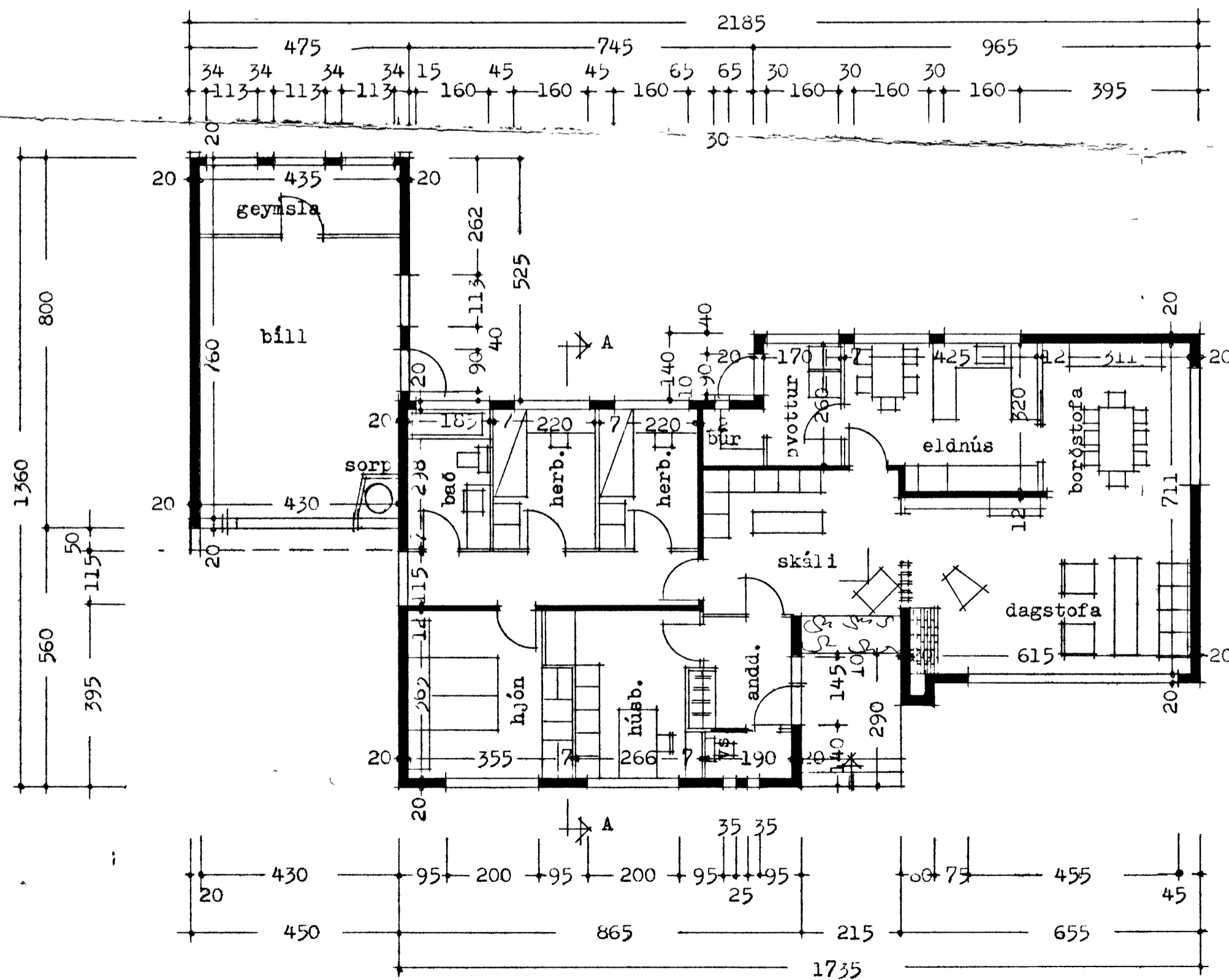
grunnmynd
