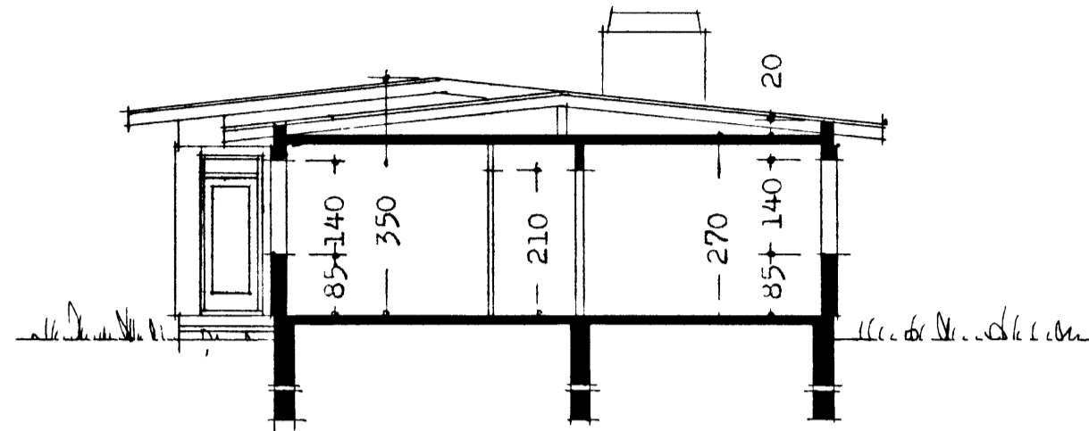
Skurður A-A
