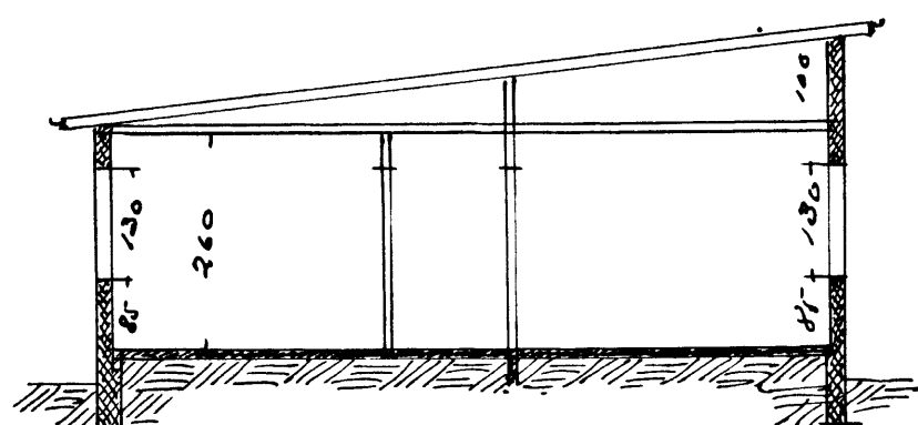
SKURÐUR
