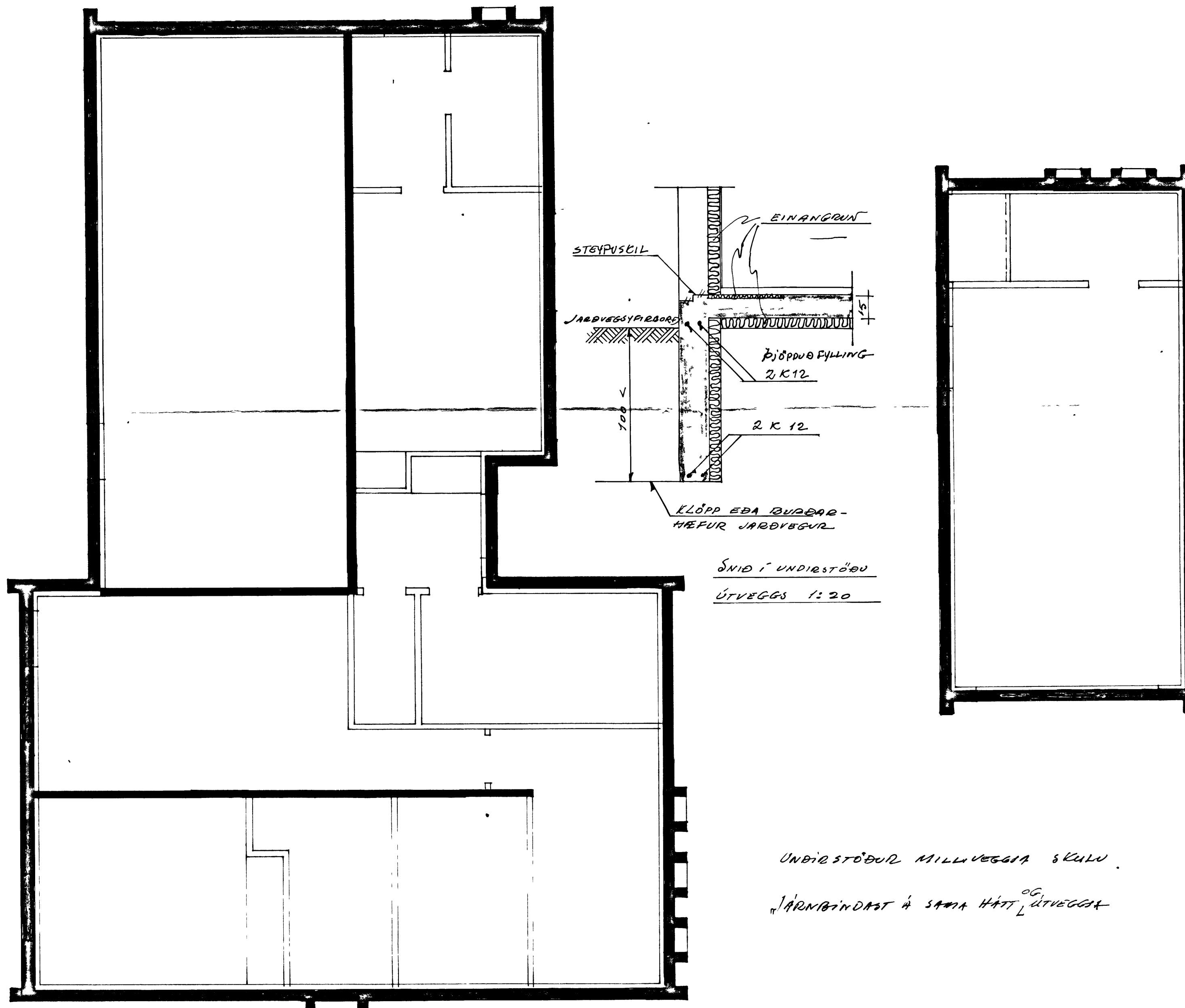
UNDIRSTÖÐUR. GRUNNMÝND 1:50
