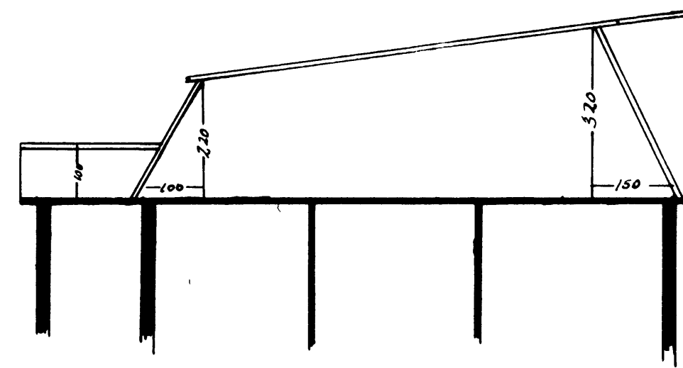
SKURÐUR
