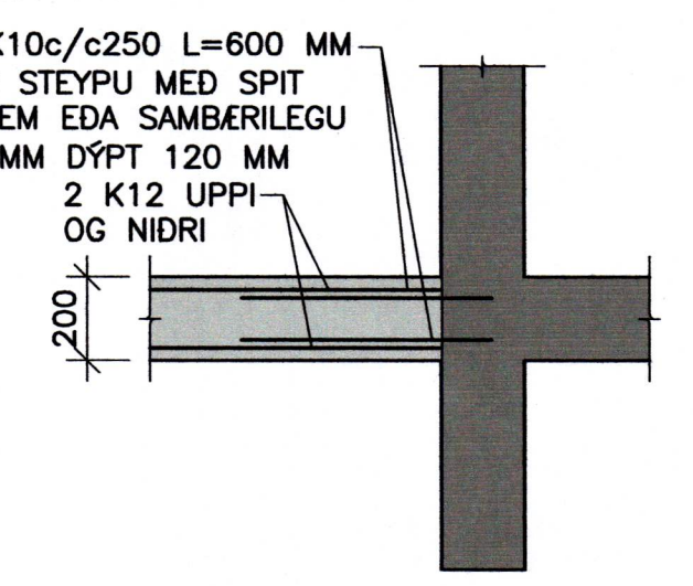
D DEILI 201 1:20
