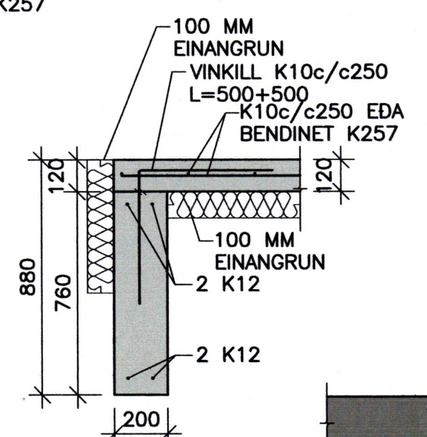
03 SNID 201 1:20
