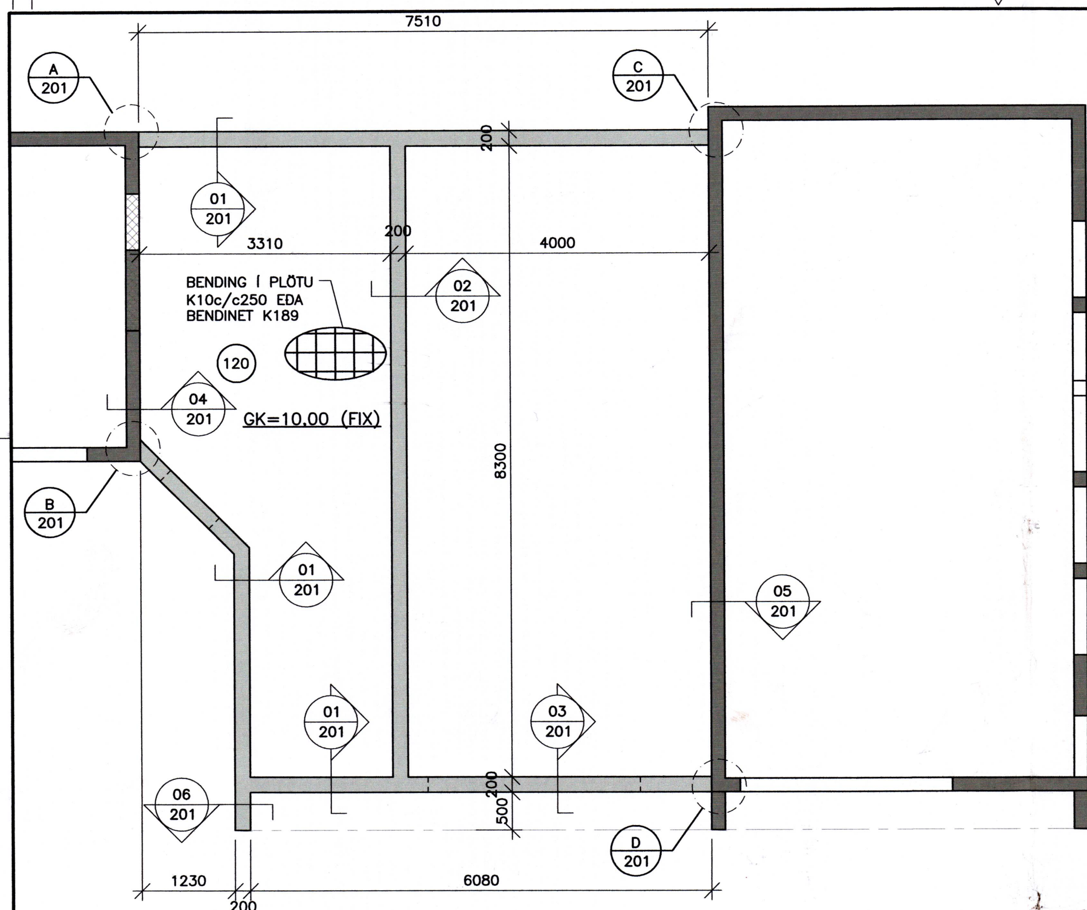
GRUNNMYND SÖKKLA. 1:50
