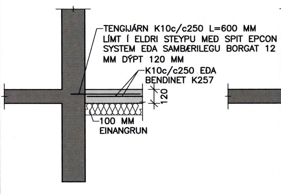
04 SNID 201 1:20
