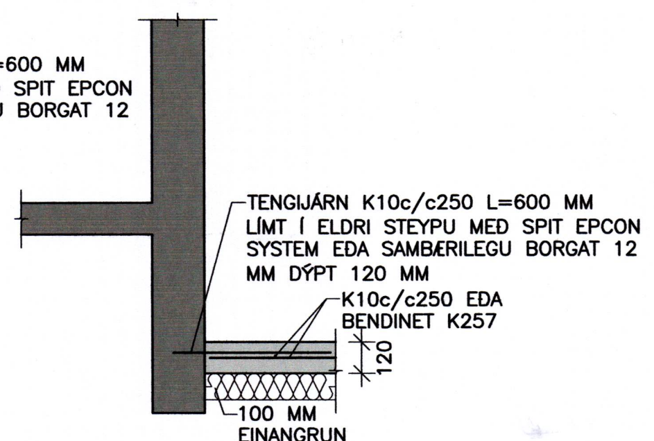
05 SNID 201 1:20
