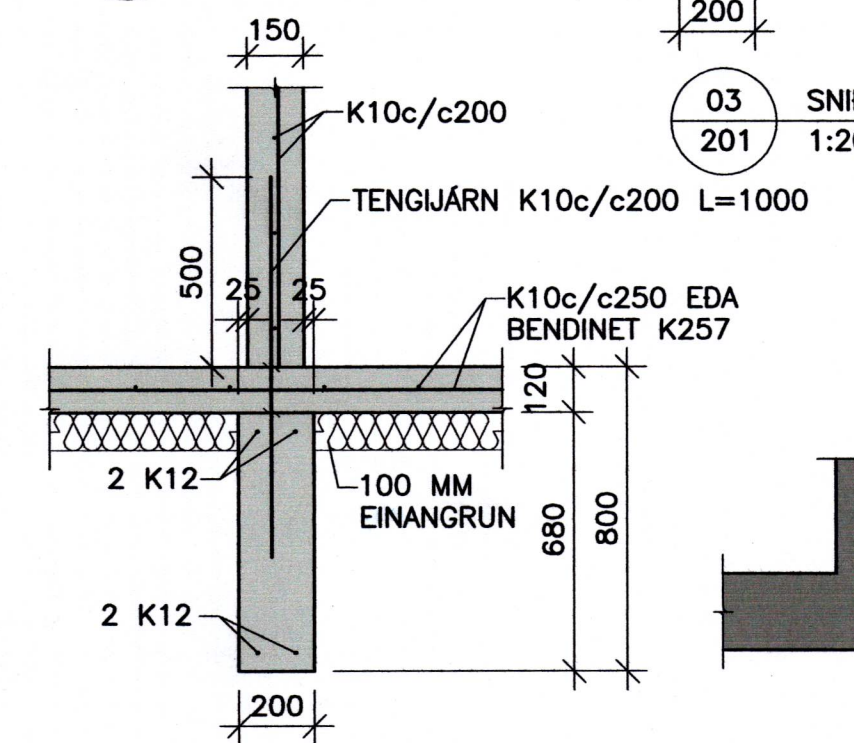
02 SNID 201 1:20
