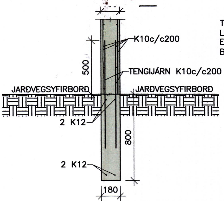
06 SNID 201 1:20
