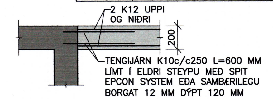
A DEILI 201 1:20
