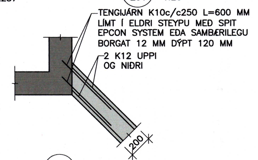
B DEILI 201 1:20
