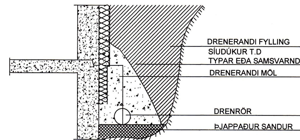
FRÁGANGUR DRENLAGNAR
