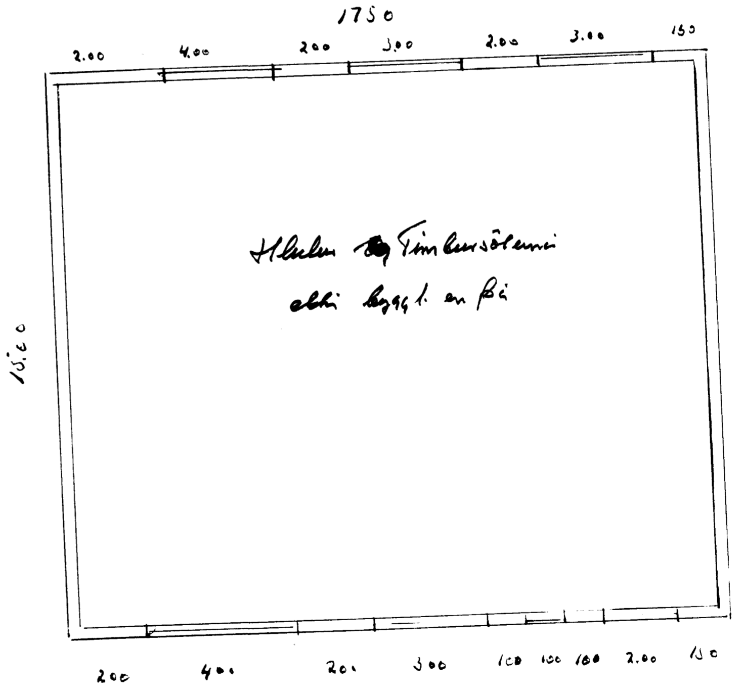
GRUNNMYND AÐRI HLIÐAR 1:100
