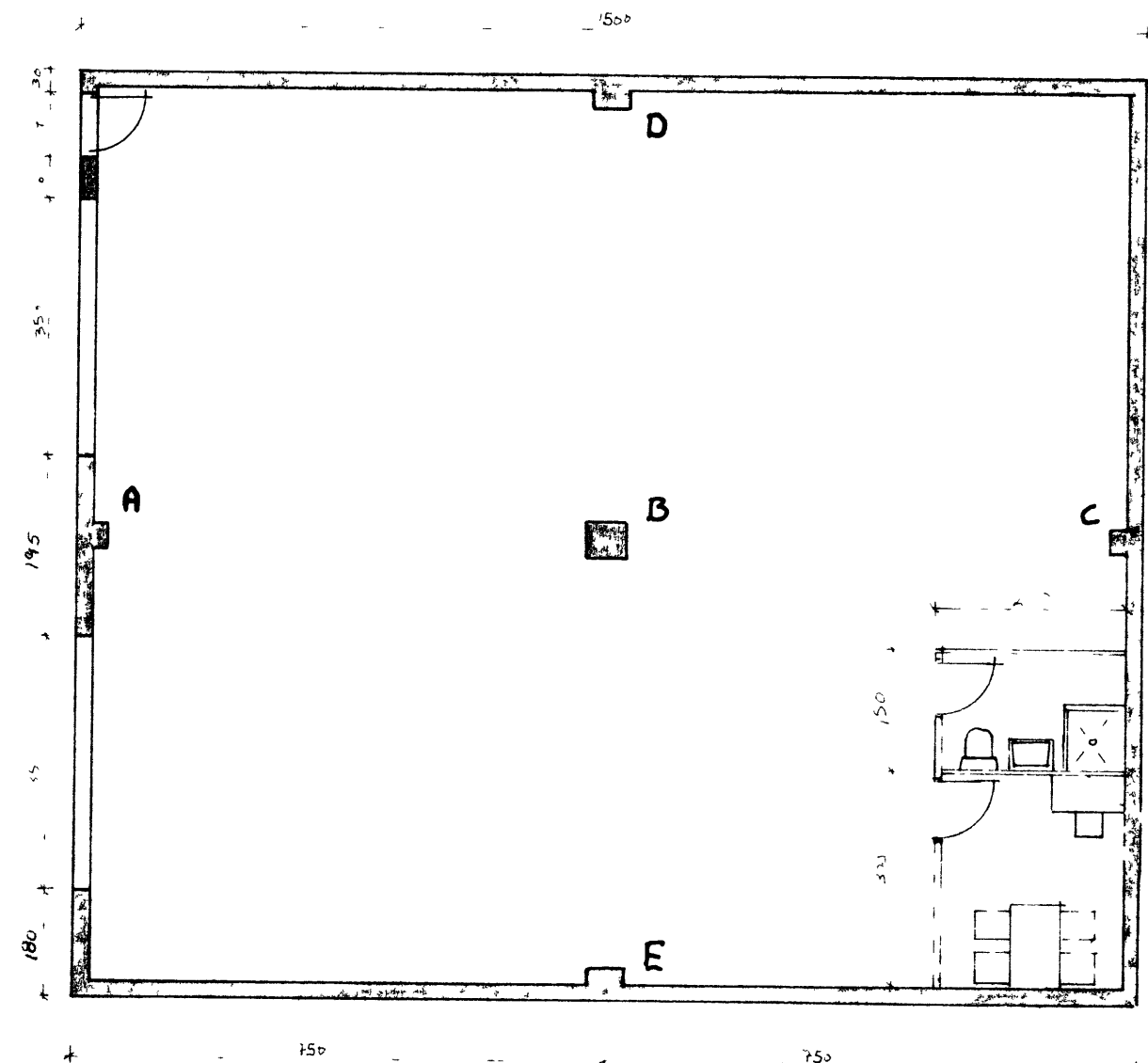
grunnmynd 1 gólf MKV 1:100
