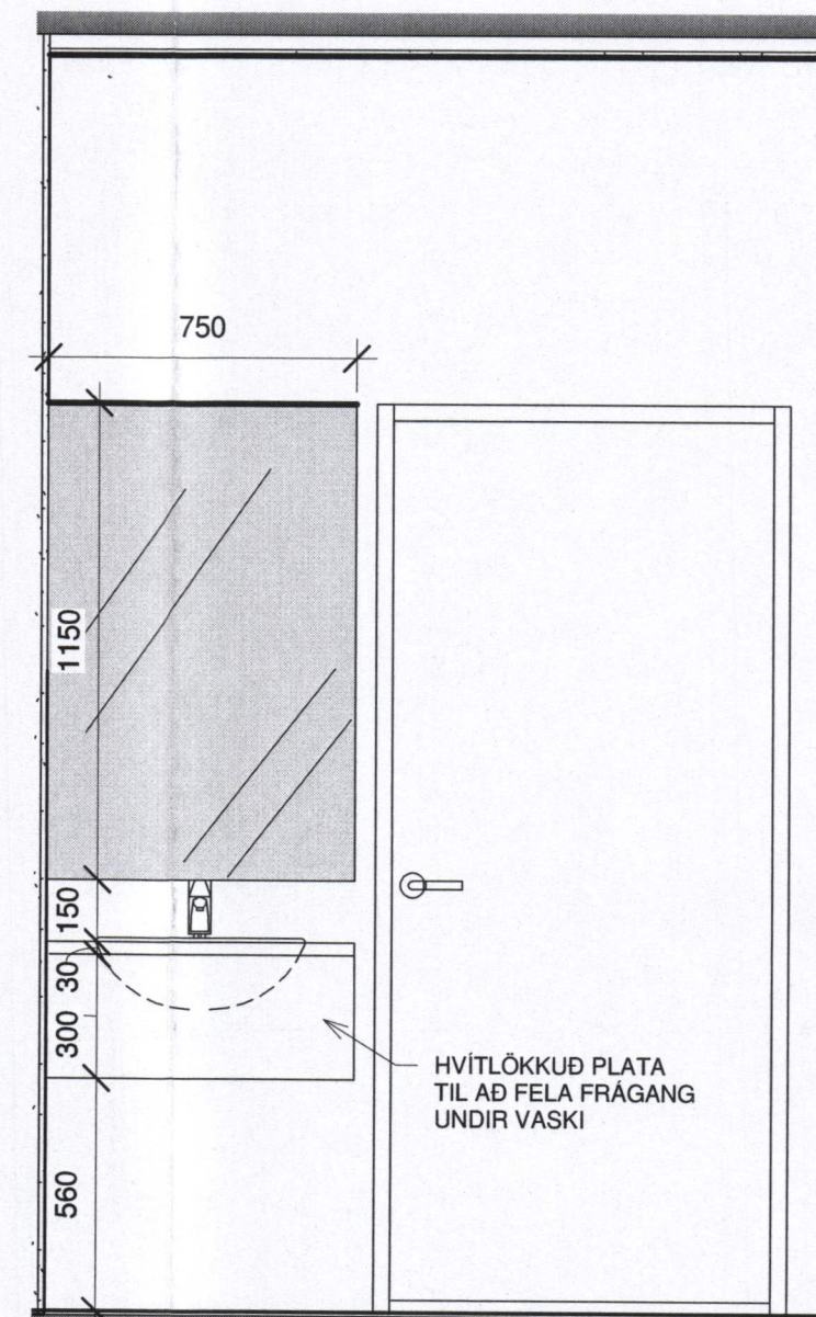
3 VS. ÁSÝND 3 1 : 20
