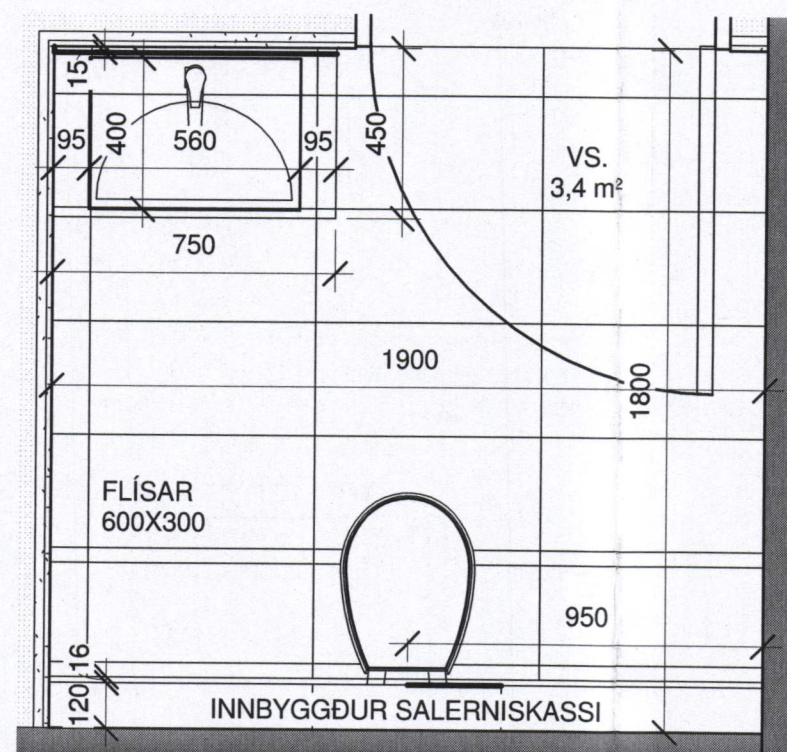
5 VS. GRUNNMYND 1 : 20
