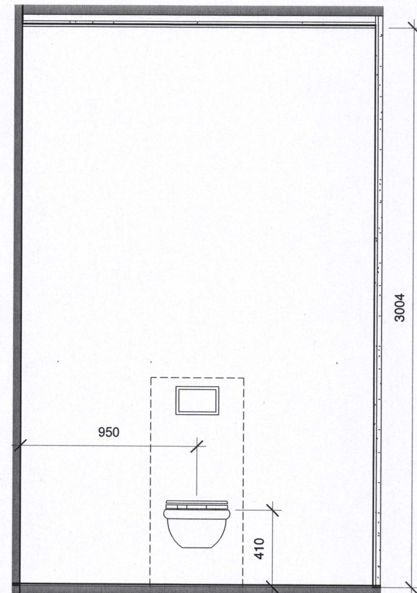
1 VS. ÁSÝND 1 1 : 20
