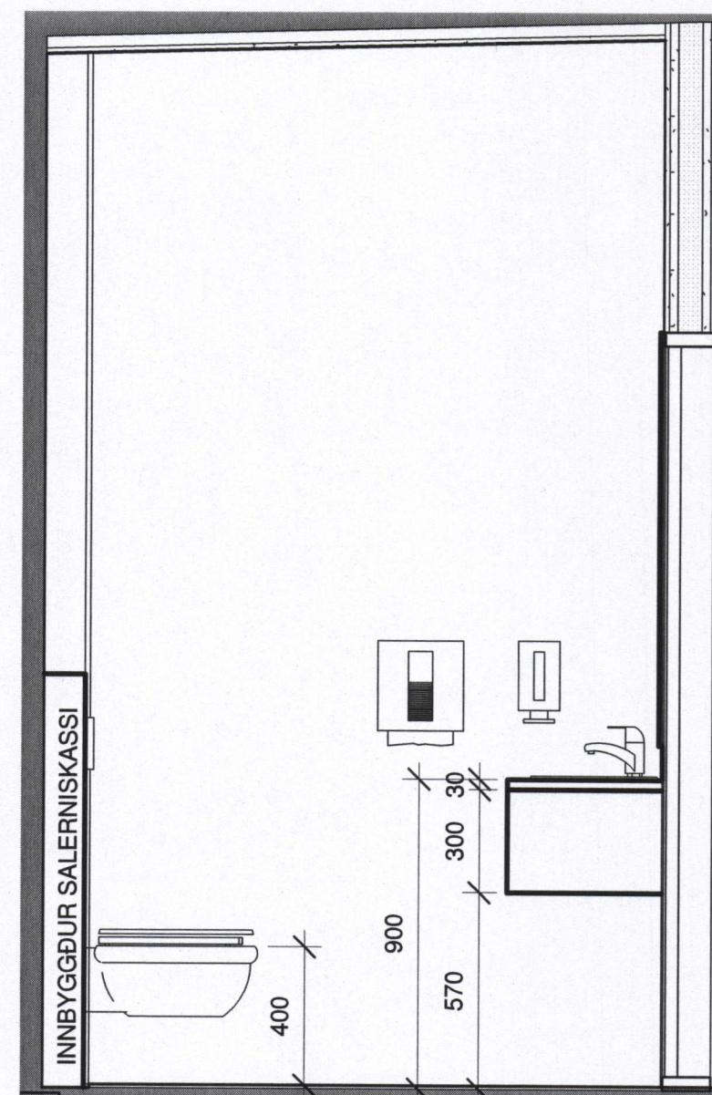
2 VS. ÁSÝND 2 1 : 20
