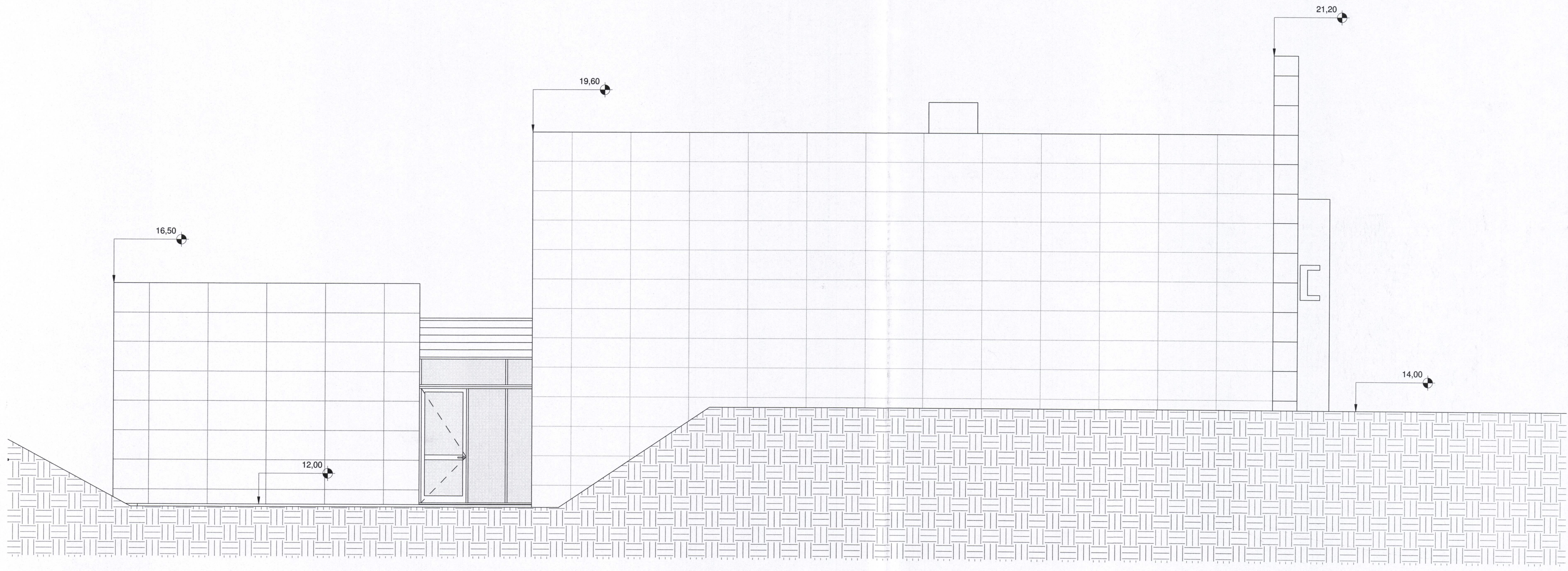
2 SUÐUR 1.50 1:50
